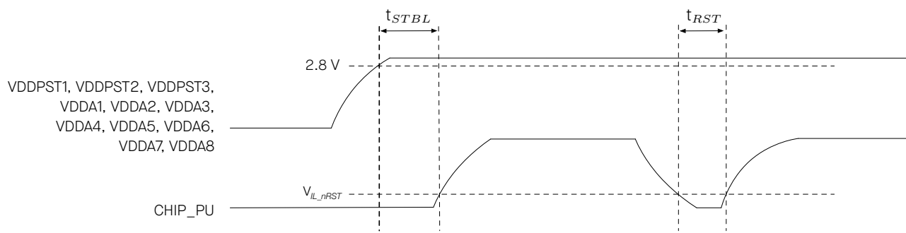
图 2-4. 上电和复位时序参数图
