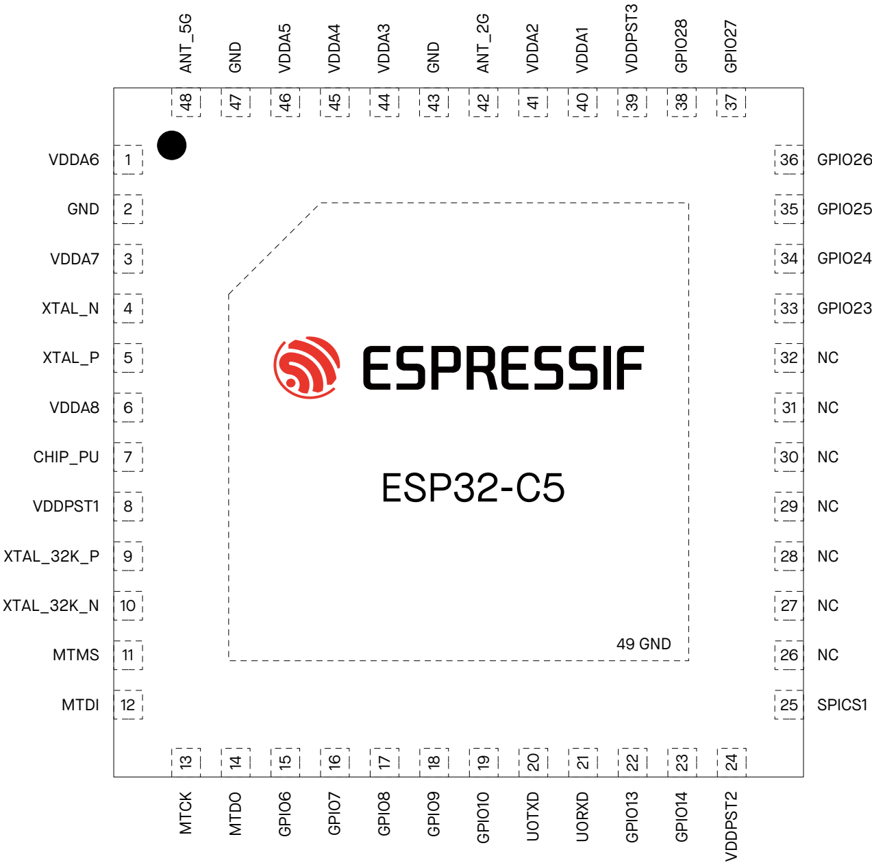
图 2-2. ESP32-C5HF4 管脚布局（俯视图）
