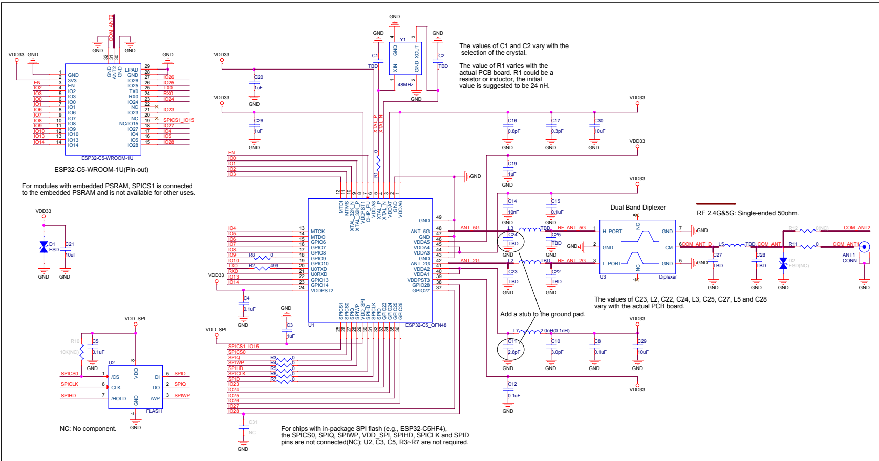
图 8-2. ESP32-C5-WROOM-1U 原理图
