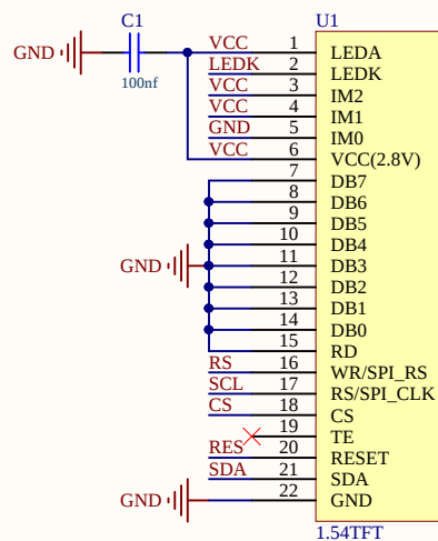
IPS屏22Pin FPC接口
