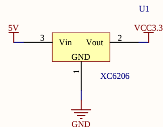
5V转3.3V电路
