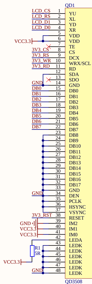
液晶屏48Pin FPC接口
