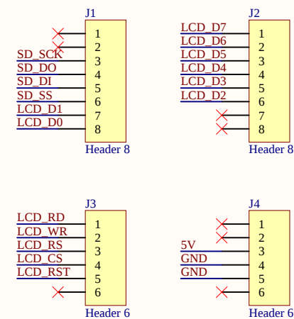
Arduino排针接口电路
