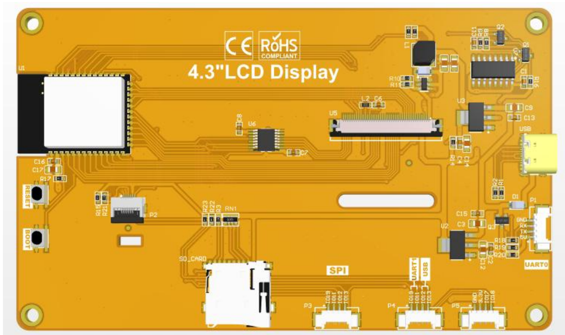
图2.1 4.3寸ESP32-S3 显示模块背面图
