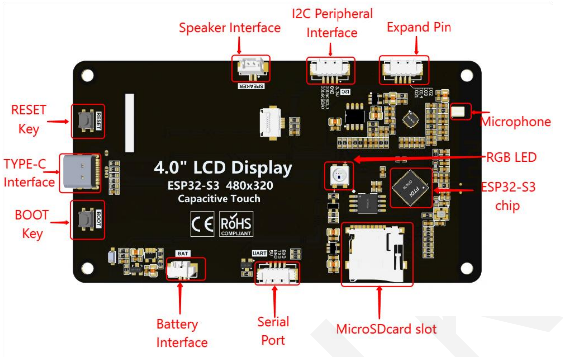
图 4.1 产品接口图
