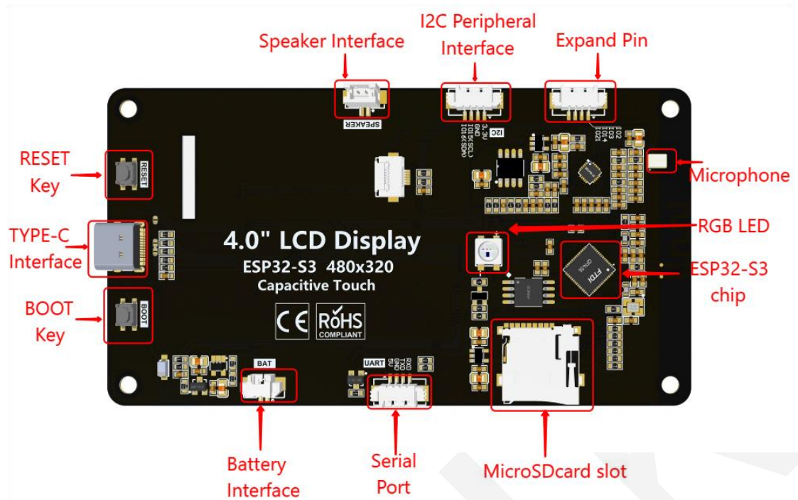
图 4.1 产品接口图
