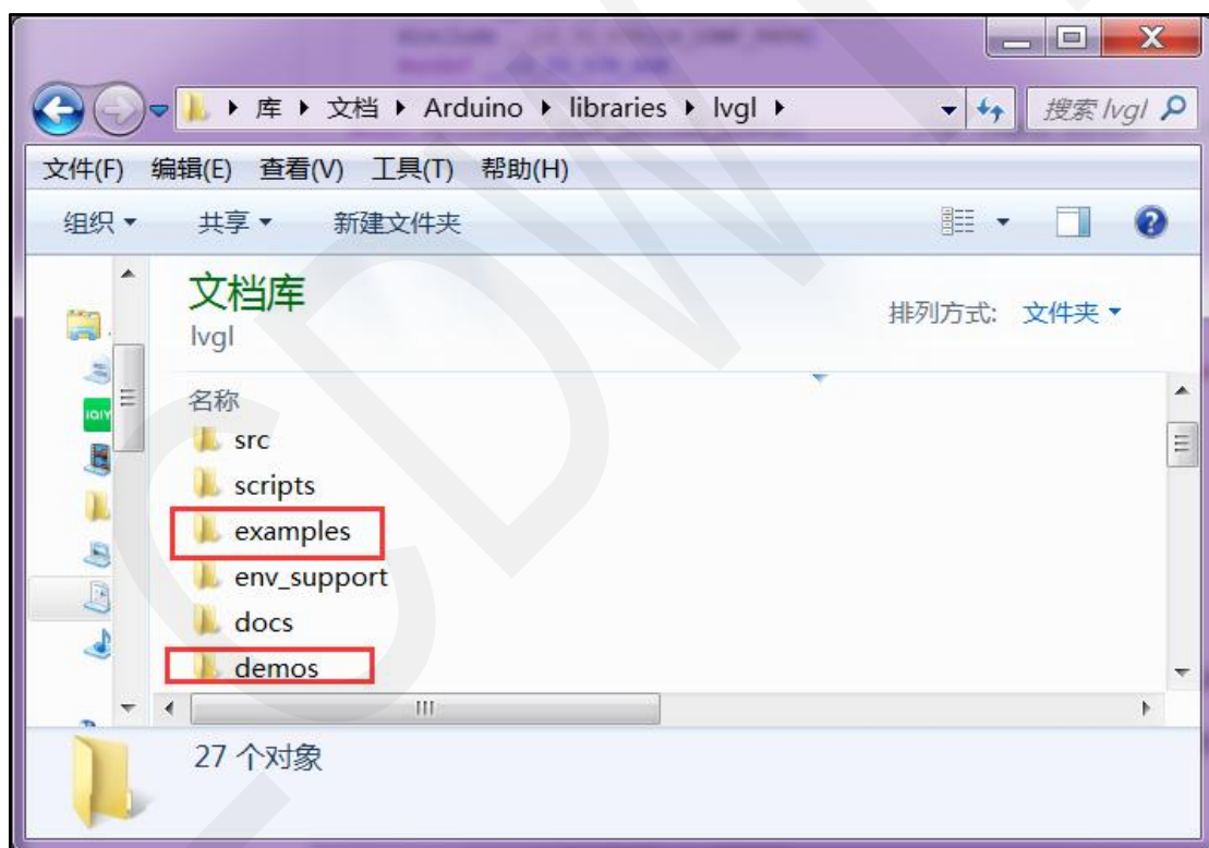
图3.6 配置LVGL库4
