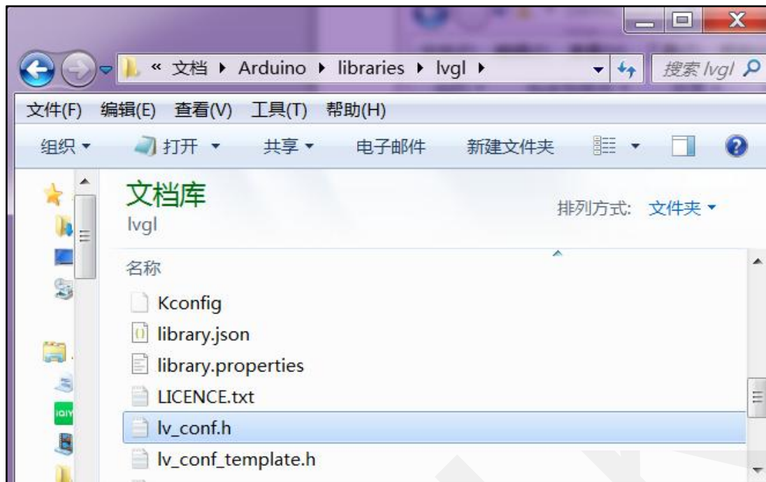
图3.3 配置LVGL库1
