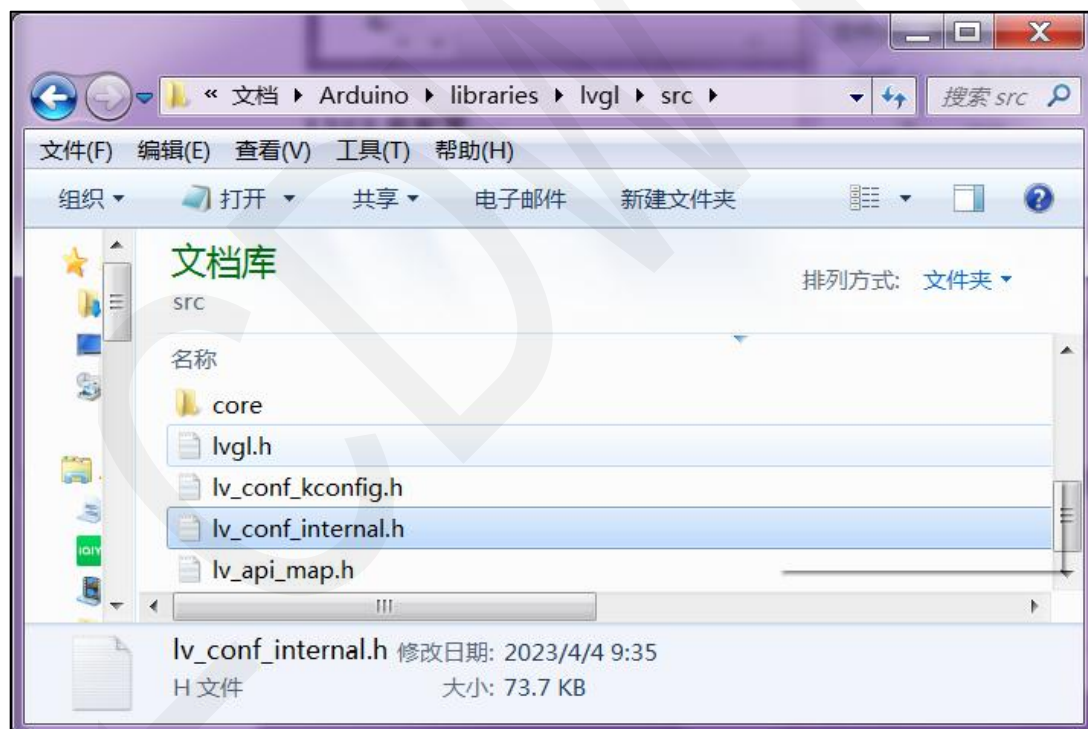
图3.4 配置LVGL库2
