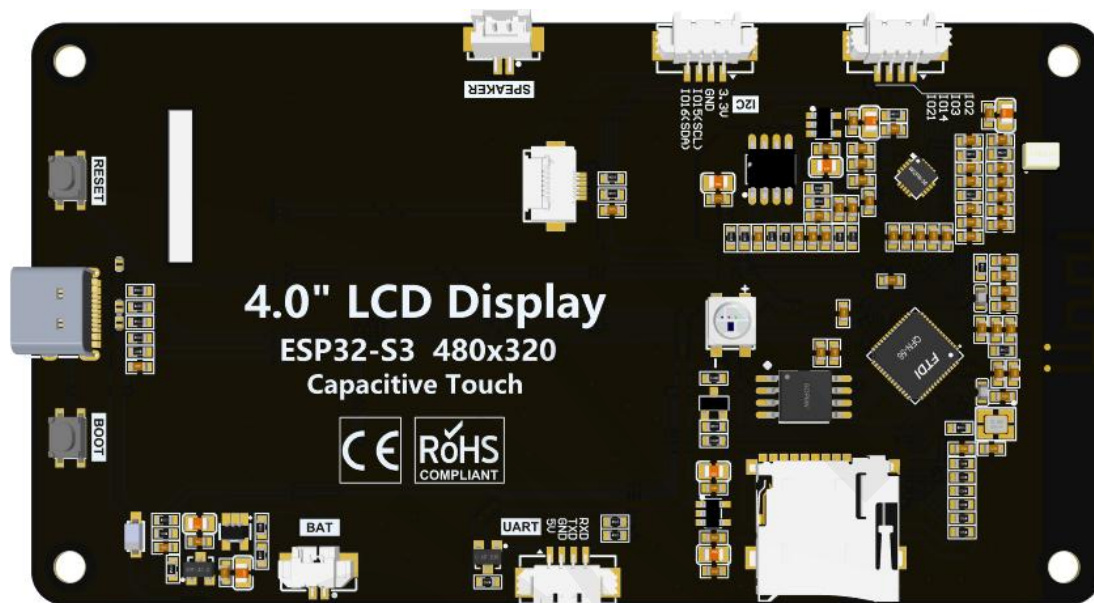
图2.1 4.0寸ESP32-S3 IPS显示模块背面图
