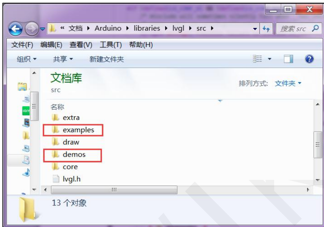
图3.7 配置LVGL库5
