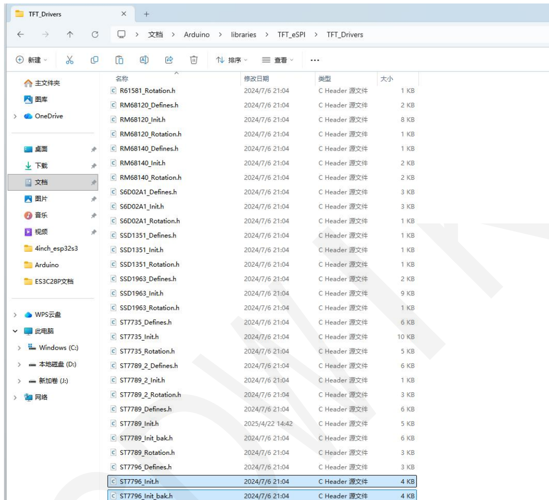
图 3.9 配置 TFT_eSPI 库 2
