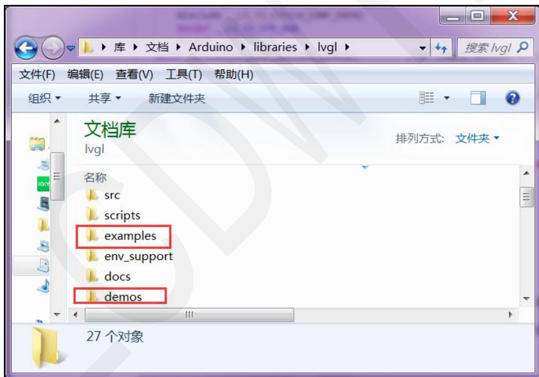
图3.6 配置LVGL库4
