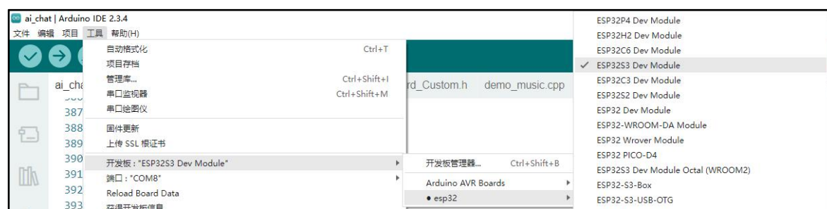
图 3.12
