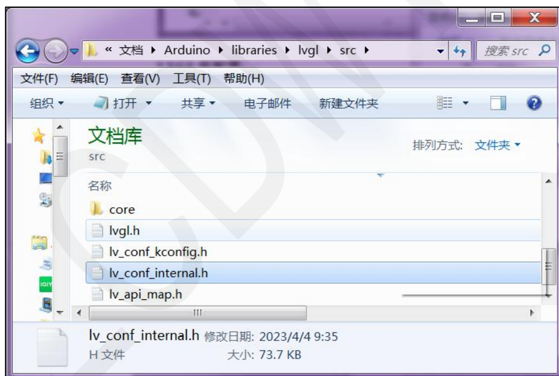
图3.4 配置LVGL库2
