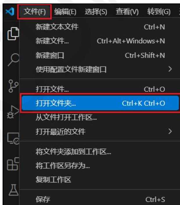
图 3.2 打开文件夹
