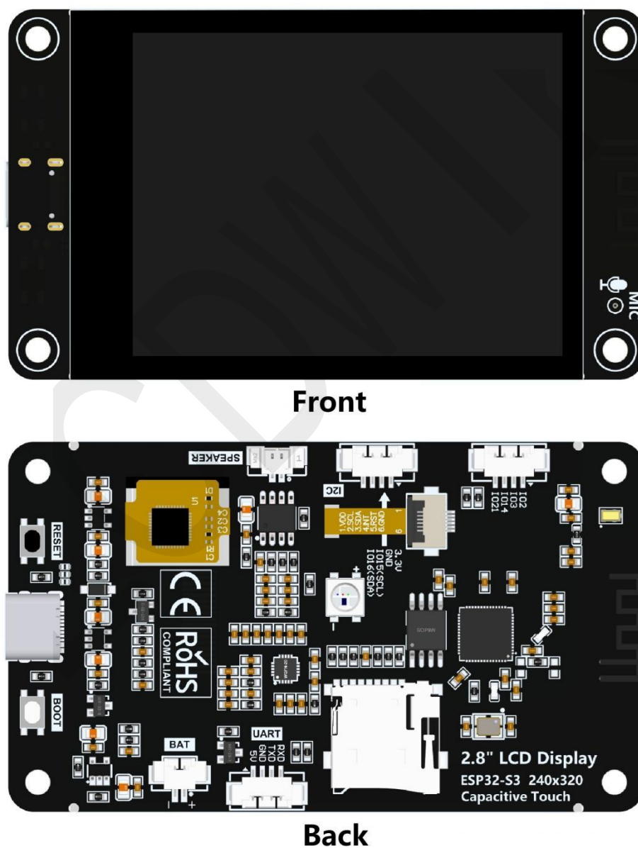
图 1.1 ES3C28P 产品图
