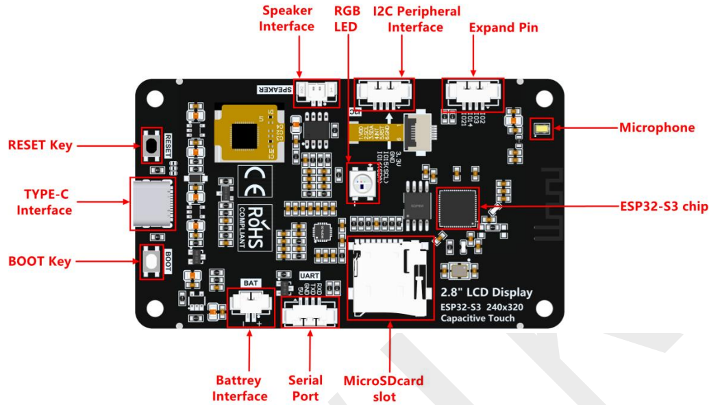
图 4.1 产品接口图
