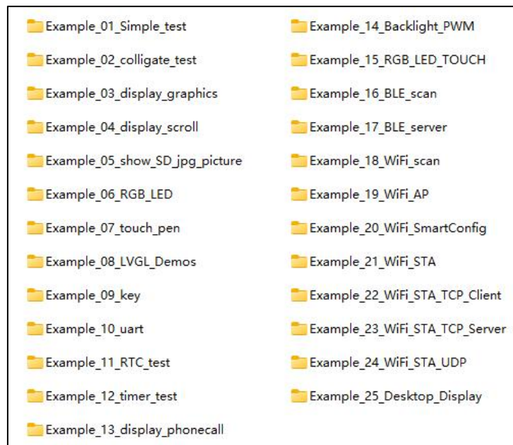
图 3.10 示例程序
