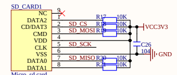
MicroSD卡槽接口电路
