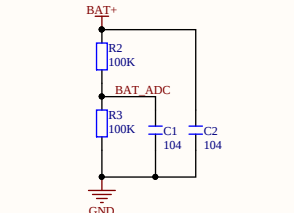
电池电量检测电路
