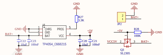
电池充放电管理电路
