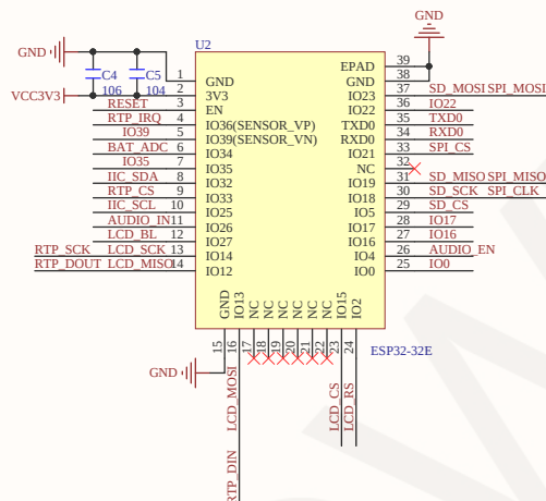
ESP32-32E主控电路
