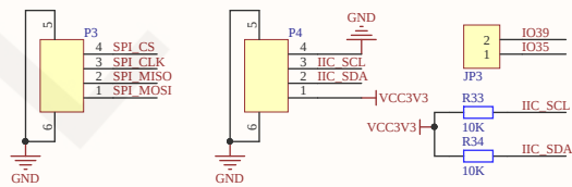
扩展IO以及外设接口电路
