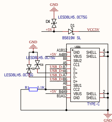
Type-C接口电路
