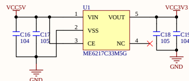
5V转3.3V稳压电路
