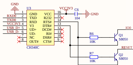
USB转串口以及一键下载电路
