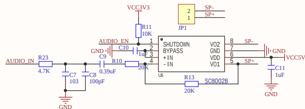
音频功放电路
