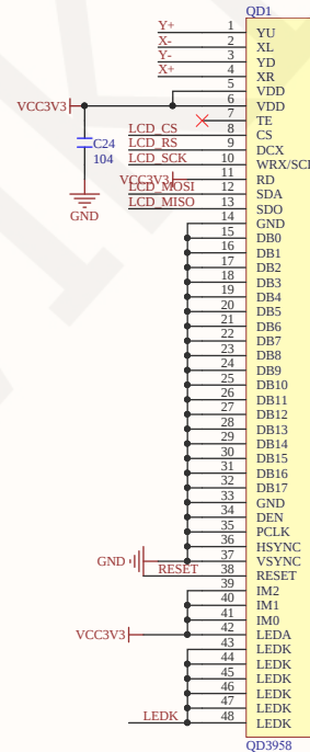
48P液晶屏排线焊接接口
