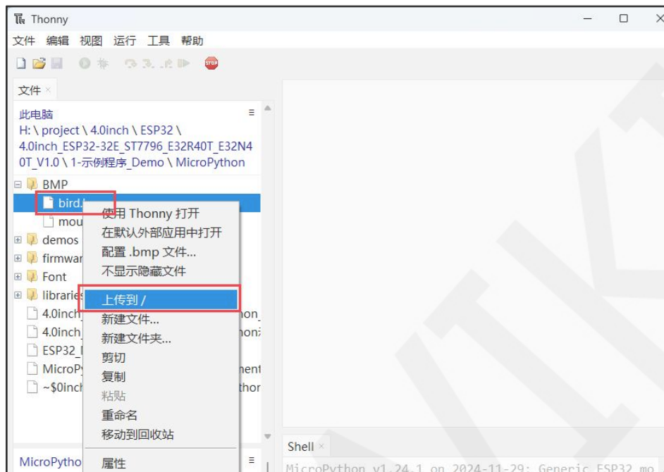
图3.4 上传文件到ESP32设备
