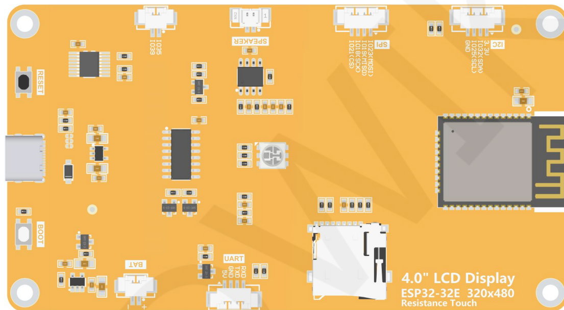
图2.1 4.0寸ESP32-32E显示模块背面图
