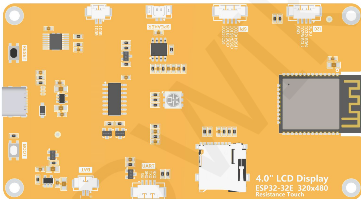
图2.1 4.0寸ESP32-32E显示模块背面图
