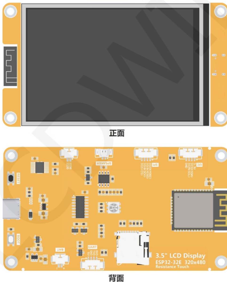
图 1.1 E32R35T 产品图
