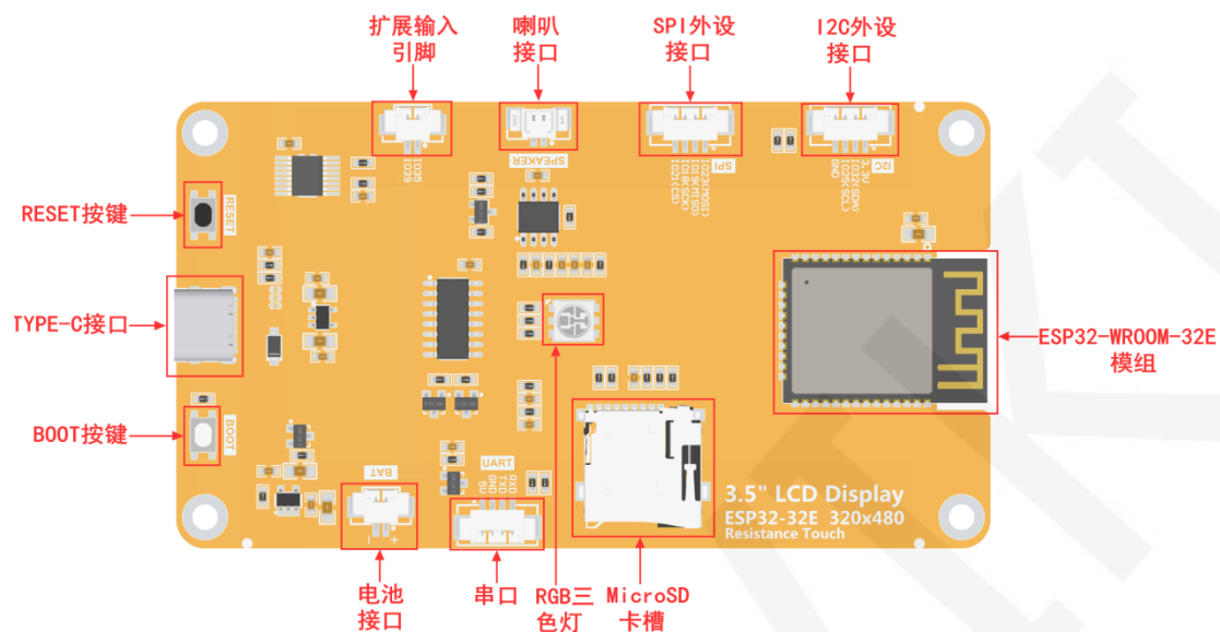
图 4.1 产品接口图
