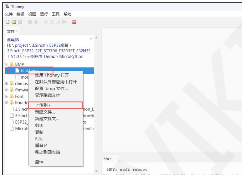
图3.4 上传文件到ESP32设备
