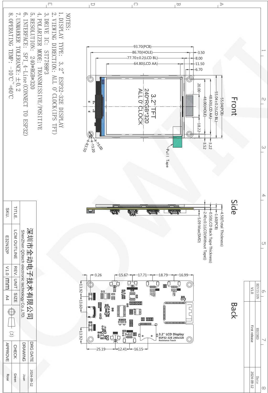
图 5.2 E32N32P 产品尺寸图
