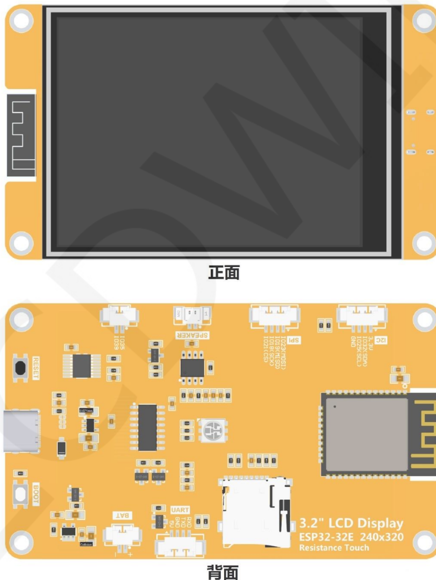
图 1.1 E32R32P 产品图
