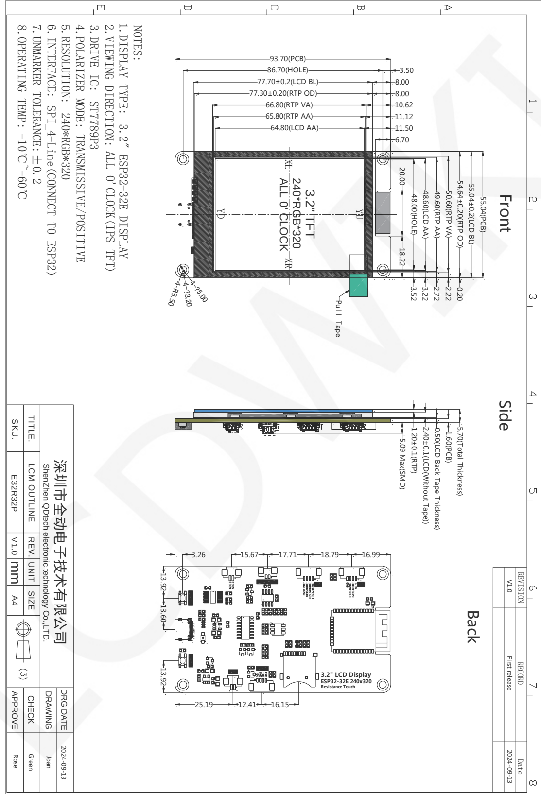
图 5.1 E32R32P 产品尺寸图
