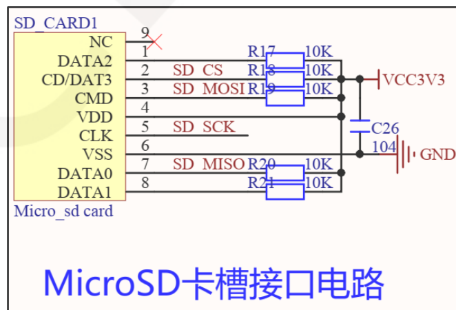
图 3.18 MicroSD 卡槽接口电路
