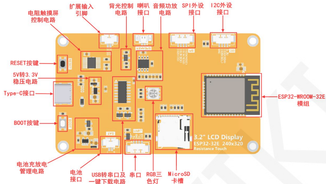
图 3.2 模块硬件资源 2
