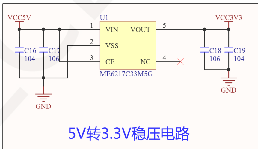
图 3.6 稳压电路
