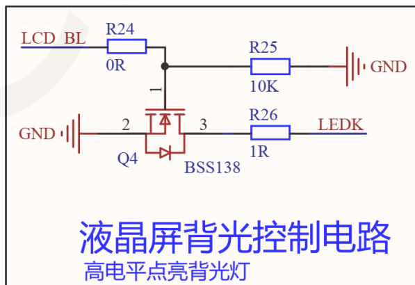
图 3.16 液晶屏背光控制电路
