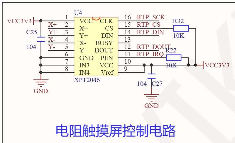
图 3.7 电阻触摸屏控制电路
