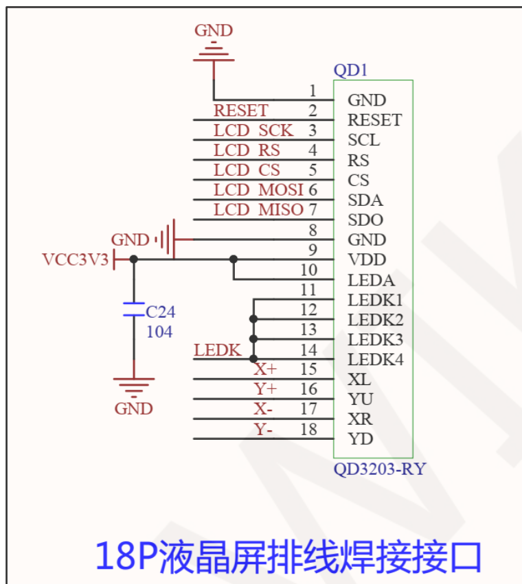
图 3.14 18P 液晶屏排线焊接接口
