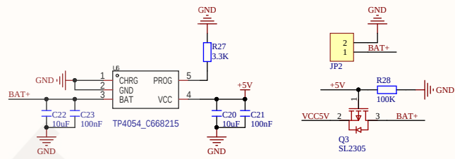
电池充放电管理电路
