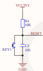
按键复位电路
