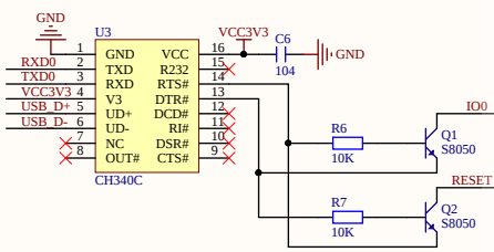
USB转串口以及一键下载电路
