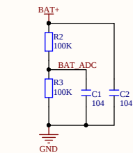
电池电量检测电路
