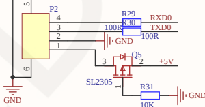
串口模块接口电路
