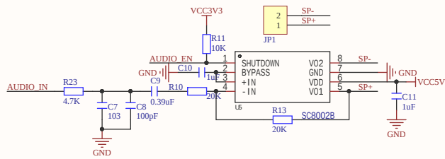
音频功放电路
