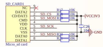
MicroSD卡槽接口电路
