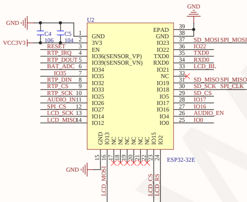
ESP32-32E主控电路
