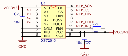
电阻触摸屏控制电路
