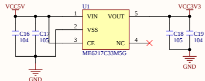
5V转3.3V稳压电路
