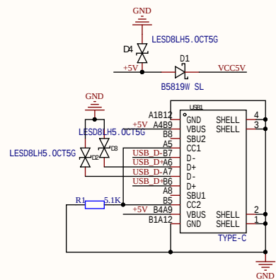
Type-C接口电路
