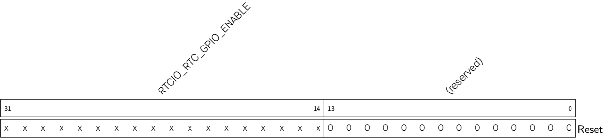
Register 4.38. RTCIO_RTC_GPIO_ENABLE_REG (0x000C)
