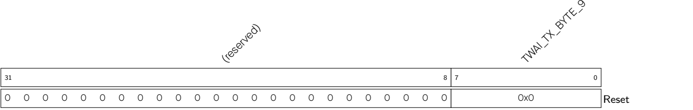
Register 21.14. TWAI_DATA_9_REG (0x0064)
