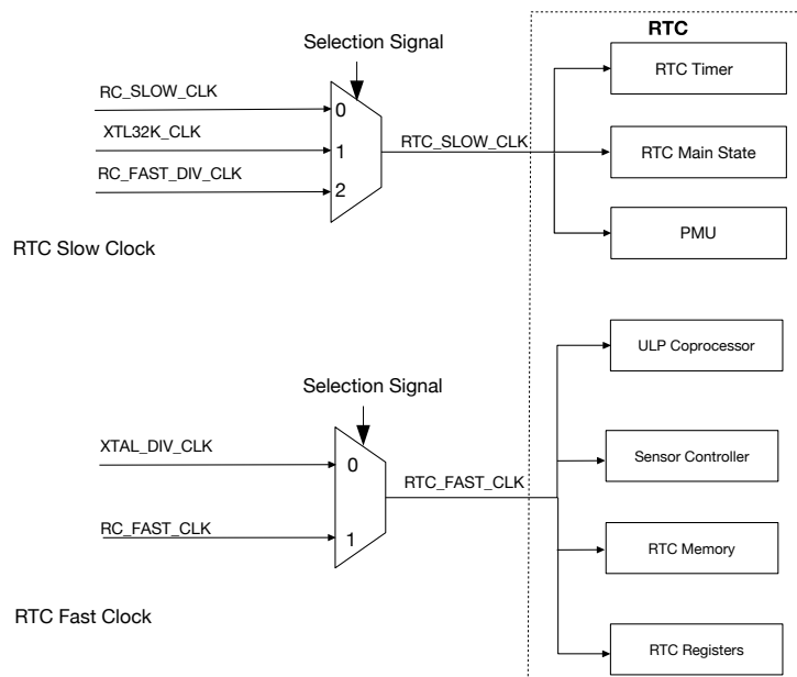
图 31-7. RTC 低功耗时钟
