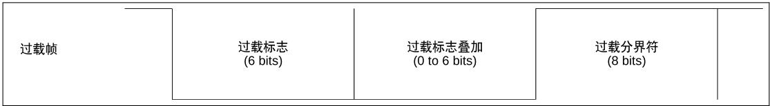
图 21-3. 过载帧中的位域
