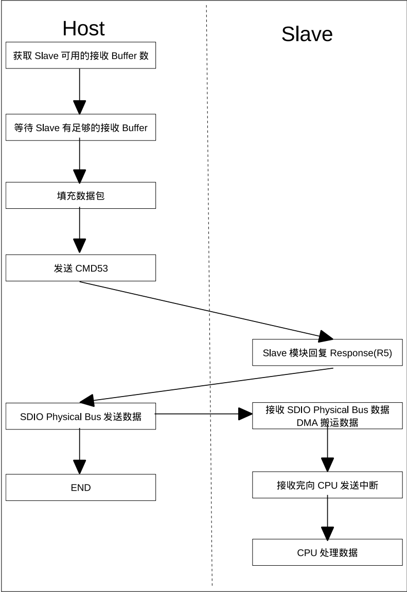
图 8-7. Slave 从 Host 接收包的流程
