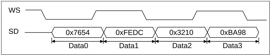
图 12-7. 第一阶段接收数据
