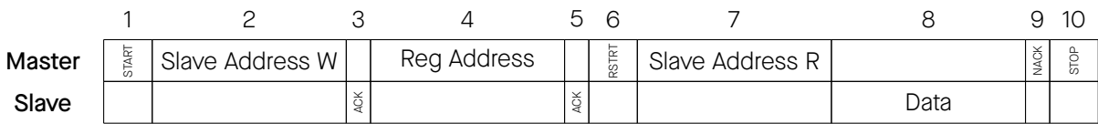
图 30-21. I2C 读操作
