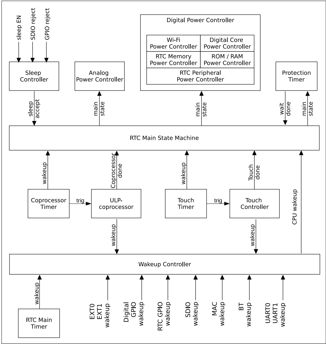
图 31-6. RTC 结构图
