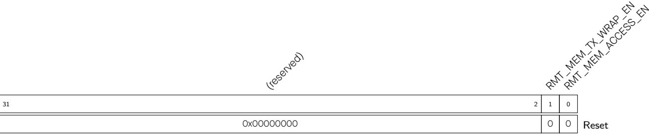
Register 15.9. RMT_APB_CONF_REG (0x00F0)
