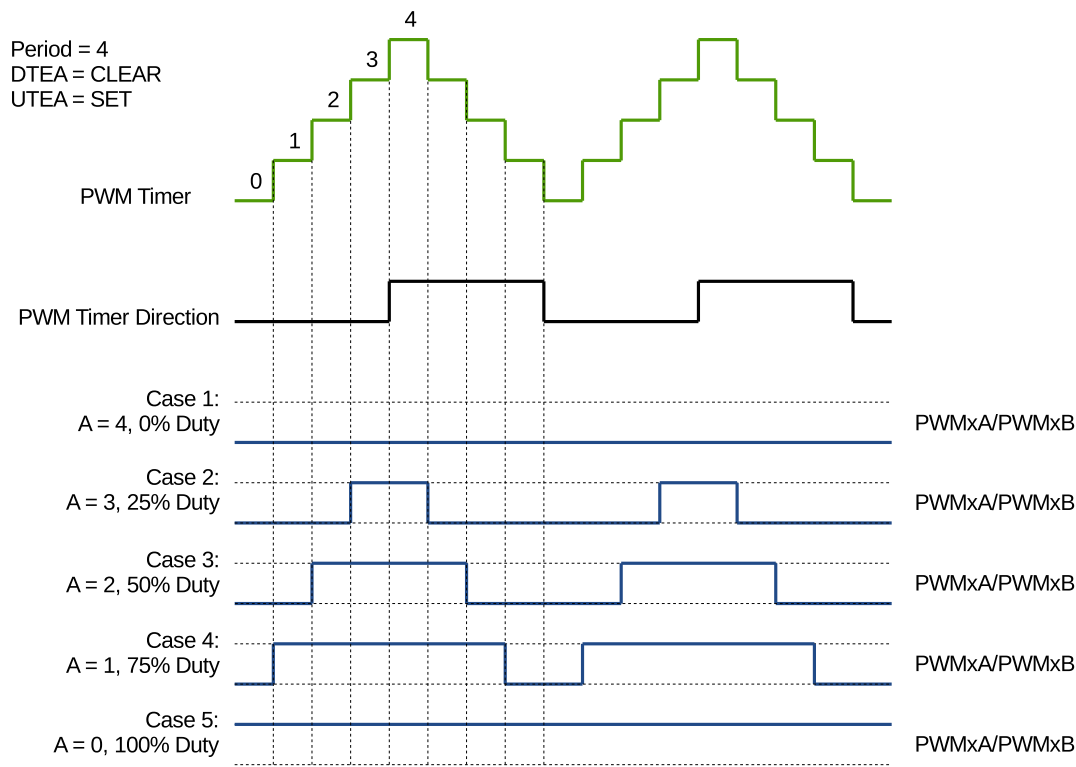
图 16-15. 递增递减模式下的对称波形
