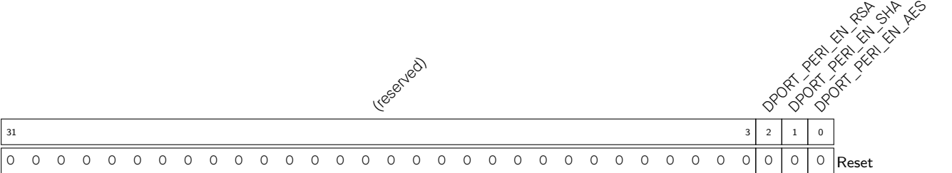
Register 5.3. DPORT_PERI_CLK_EN_REG (0x01C)
