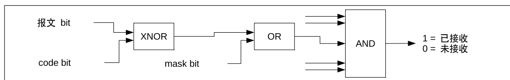
图 21-7. 接收滤波器
