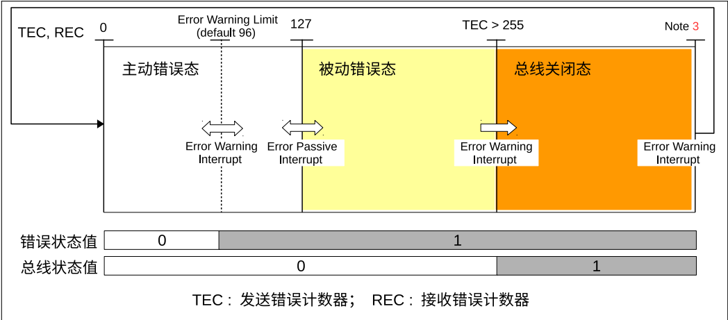
图 21-10. 错误状态变化
