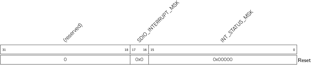
Register 9.18. MINTSTS_REG (0x0040)
