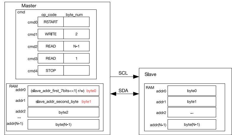
图 11-10. I2C Master 读 10-bit 地址 Slave
