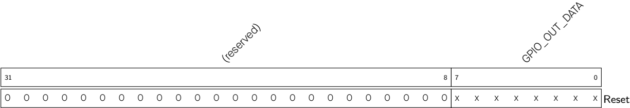
Register 4.6. GPIO_OUT1_WITC_REG (0x0018)
