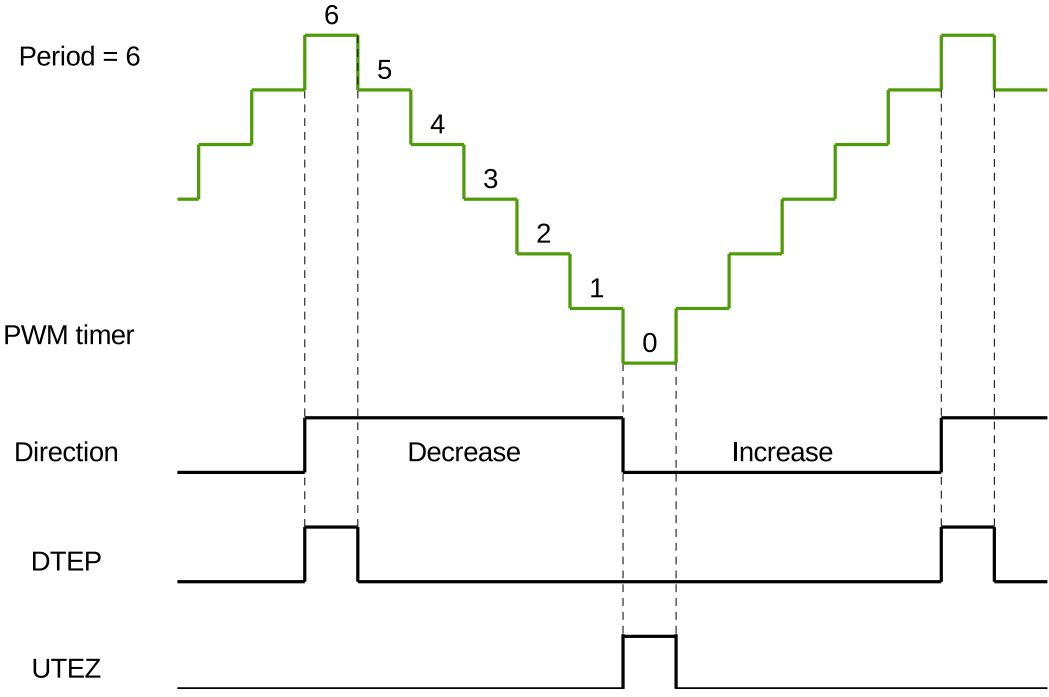
图 16-13. 递增递减模式中生成的 DTEP 和 UTEZ
