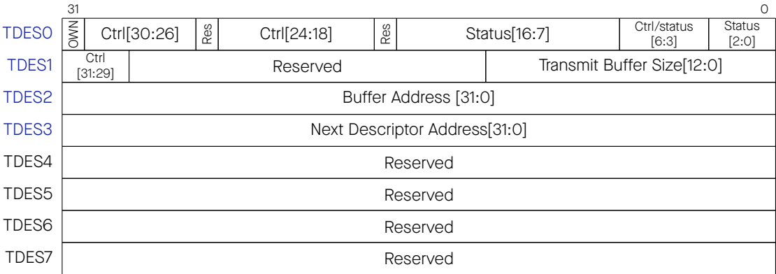
图 10-9. 发送描述符
