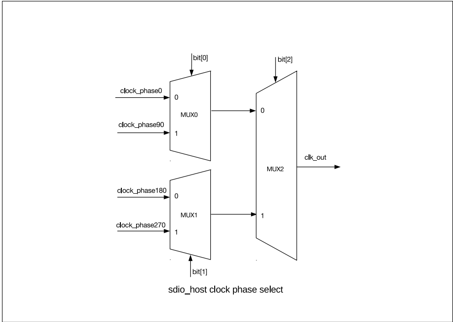
图 9-10. 时钟相位选择
