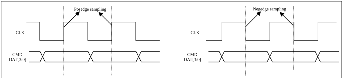
图 8-9. 采样时序图
