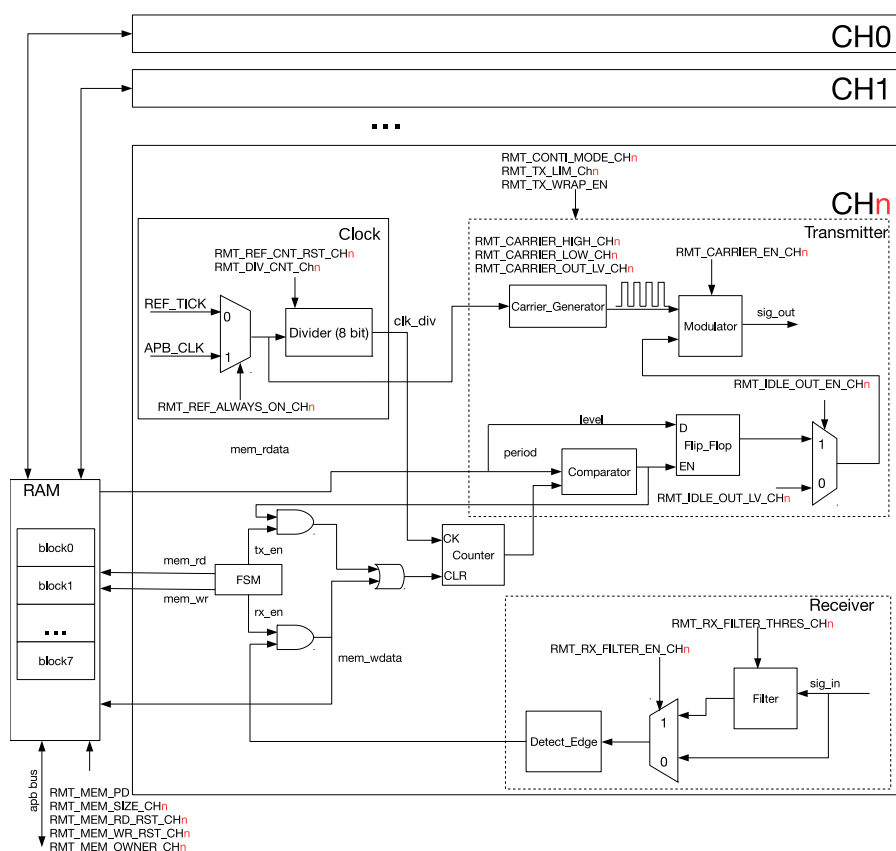
图 15-1. RMT 架构
