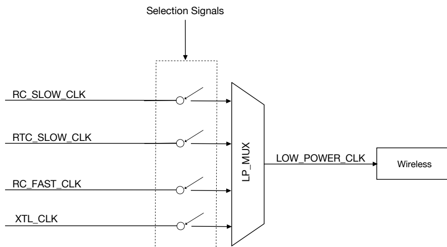
图 31-8. 数字低功耗时钟
