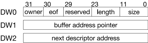
图 6-2. 链表结构图
