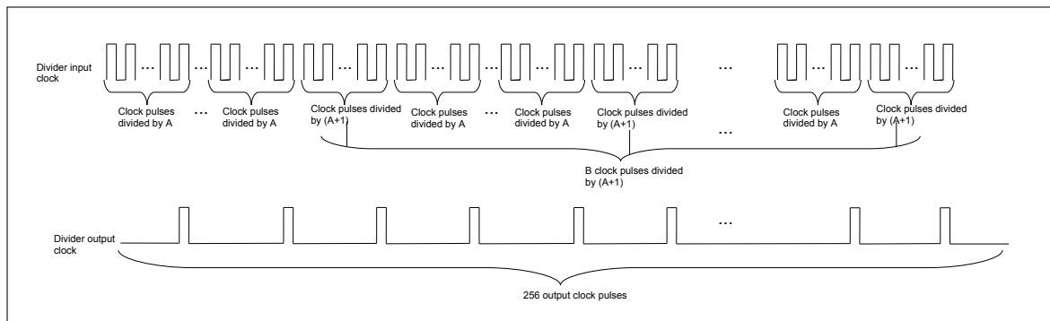
图 14-3. LED_PWM 分频器
