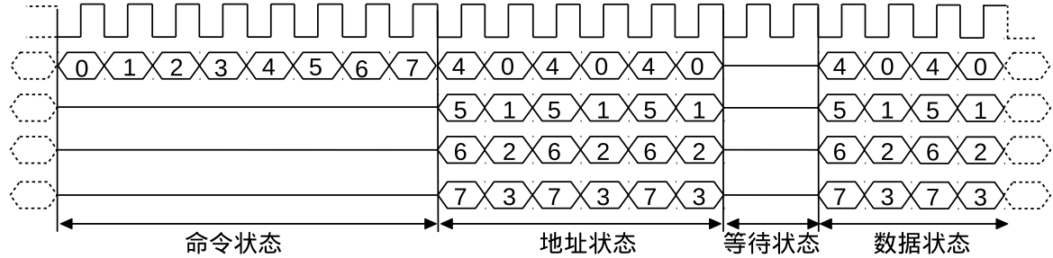
图 7-6. 并行 QSPI 接口的通信模式
