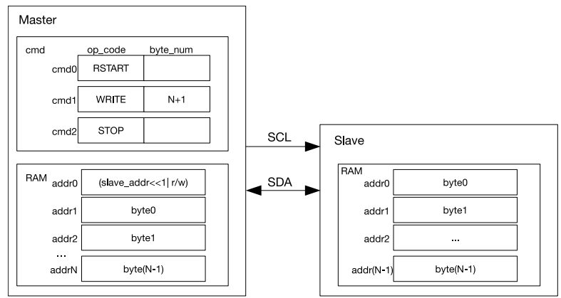
图 11-5. I2C Master 写 7-bit 地址 Slave
