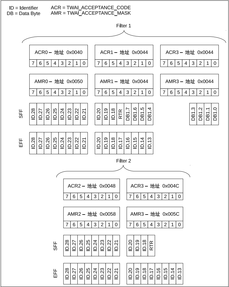
图 21-9. 双滤波模式
