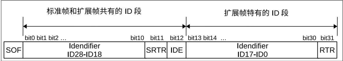
图 21-11. 丢失仲裁的 bit 位置
