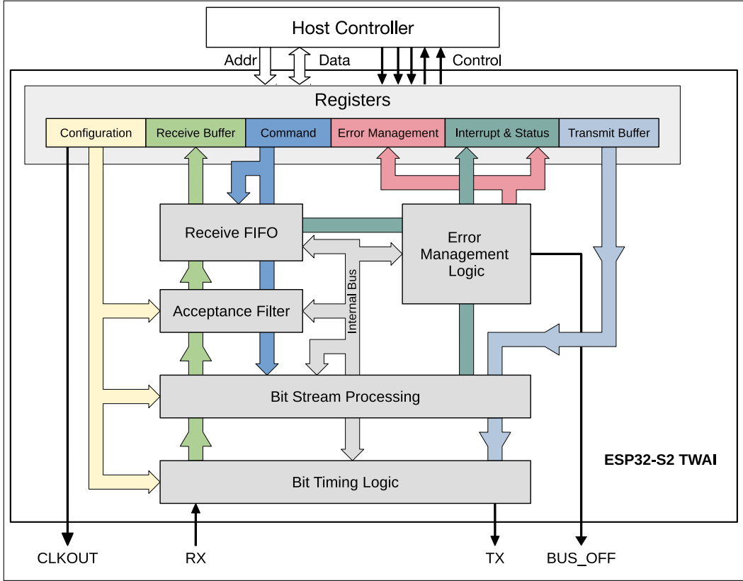
图 21-6. TWAI 概略图
