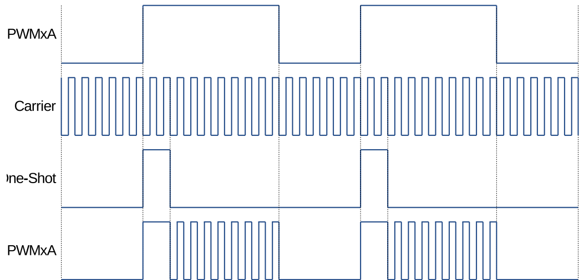
图 16-28. 载波模块的第一个脉冲和之后持续的脉冲示例
