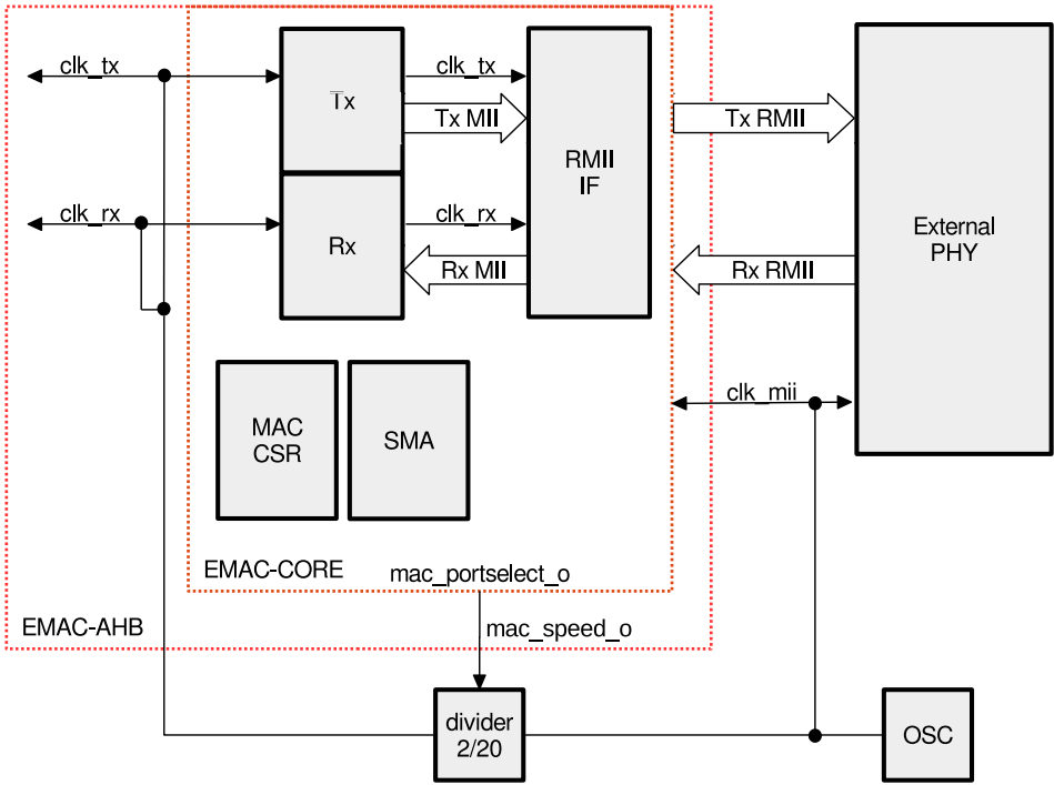
图 10-6. RMII 时钟
