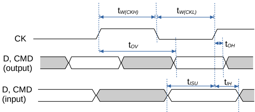
图 9-9. HS 模式下 SD/MMC 时序图
