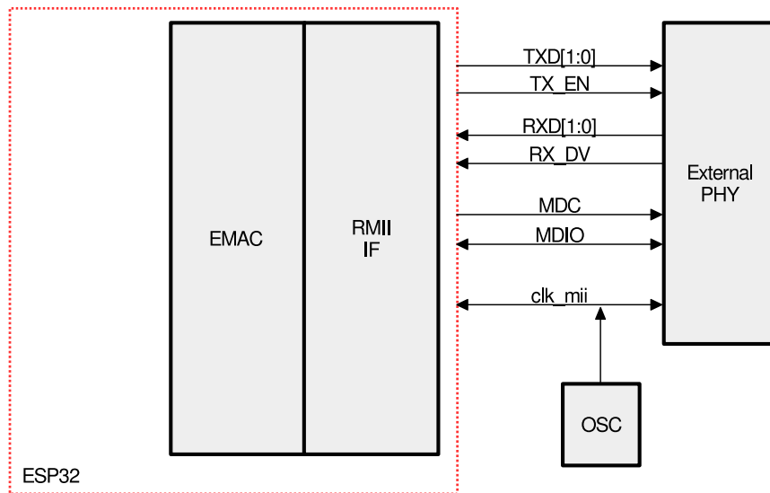
图 10-5. RMII 接口
