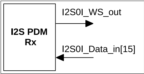
图 12-11. PDM 接收信号
