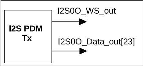
图 12-10. PDM 发送信号
