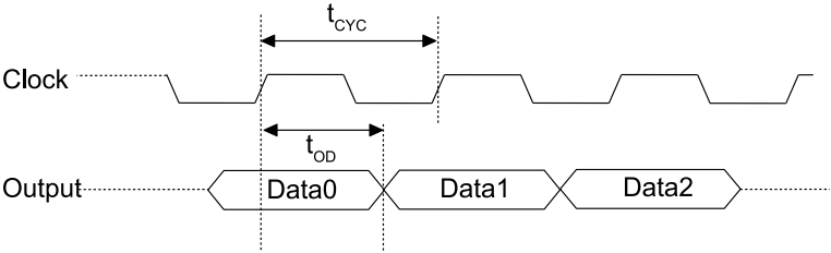
图 10-8. 发送数据时序图
