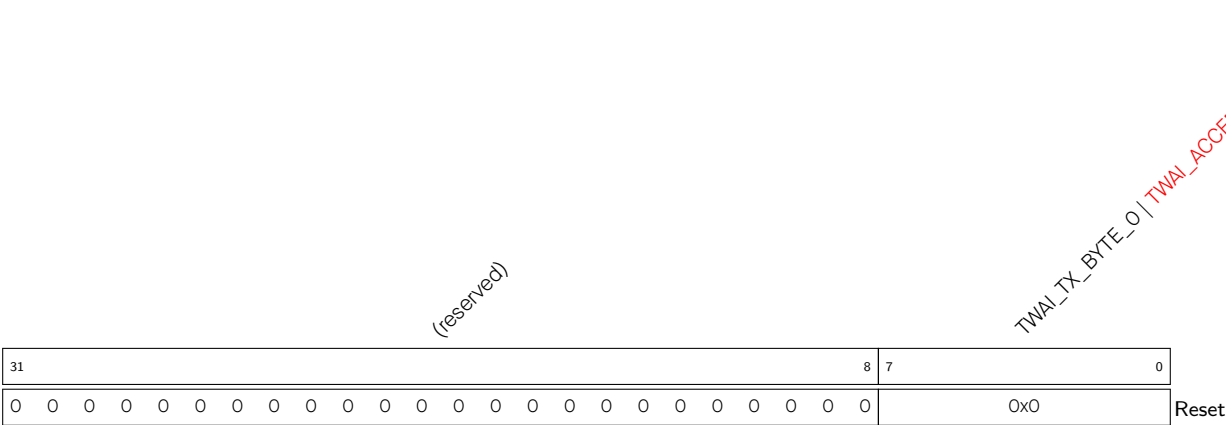
Register 21.5. TWAI_DATA_0_REG (0x0040)
