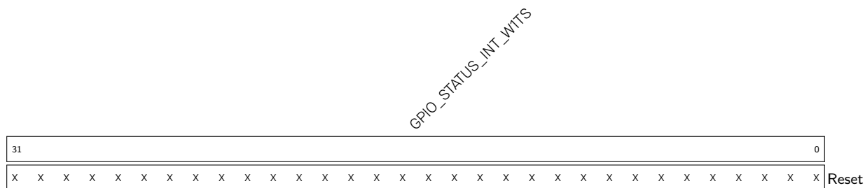
Register 4.17. GPIO_STATUS_W1TS_REG (0x0048)
