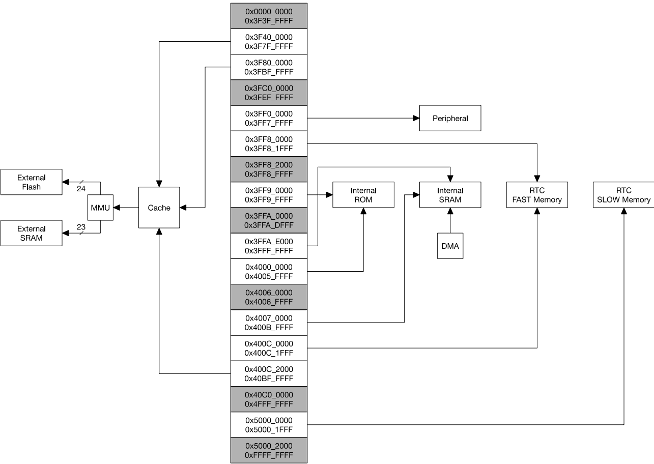
图 1-2. 地址映射结构
