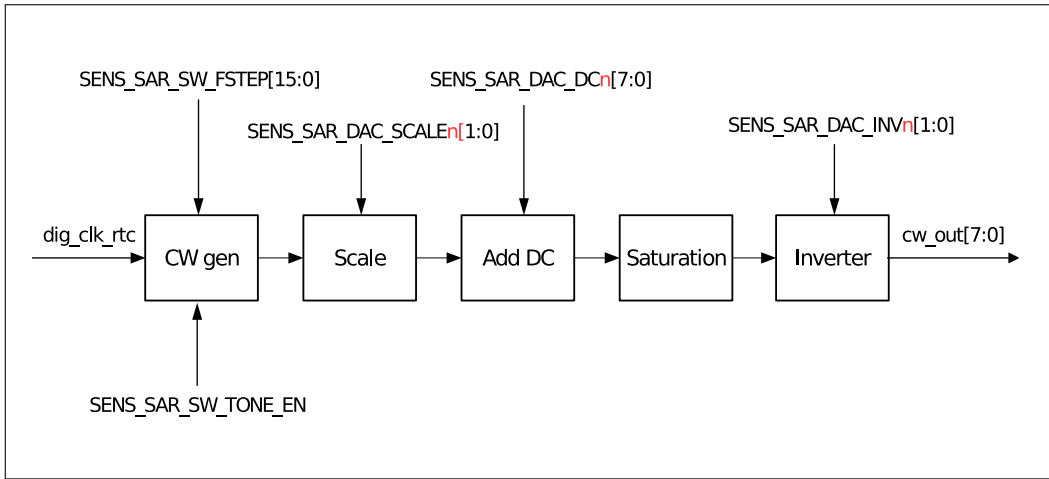
图 29-10. 余弦波形生成器的工作流程
