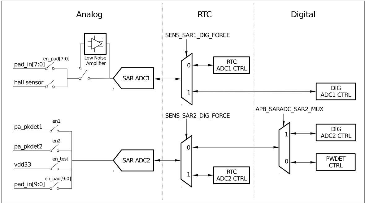
图 29-6. SAR ADC 的功能概况
