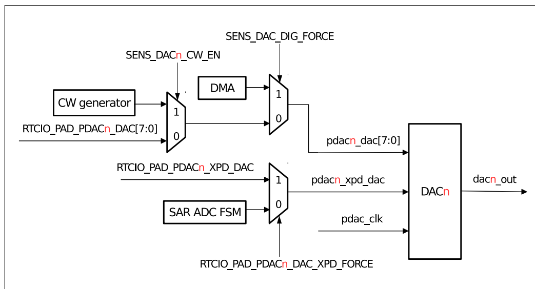
图 29-9. DAC 的功能概况
