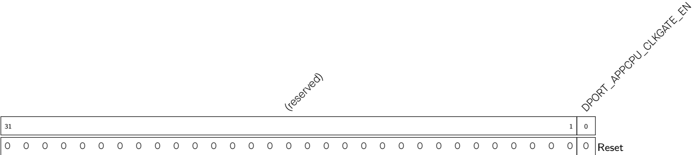
Register 5.6. DPORT_APPCPU_CTRL_REG_B_REG (0x030)
