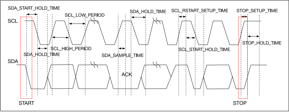
图 11-3. I2C 时序图
