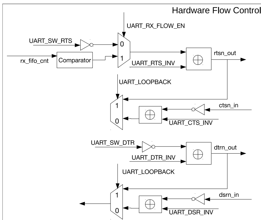
图 13-5. 硬件流控图
