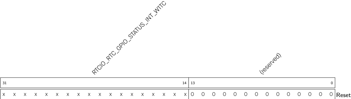
Register 4.43. RTCIO_RTC_GPIO_STATUS_WITC_REG (0x0020)
