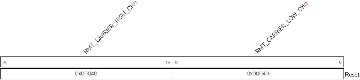
Register 15.7. RMT_CH n CARRIER_DUTY_REG ( n : 0-7) (0x00B0+4* n )
