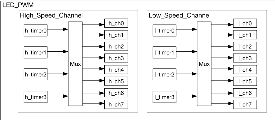
图 14-1. LED_PWM 架构
