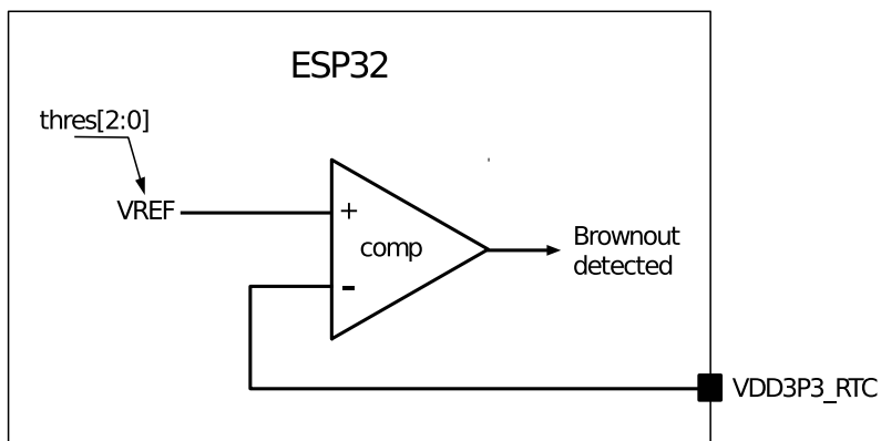
图 31-5. 欠压检测器
