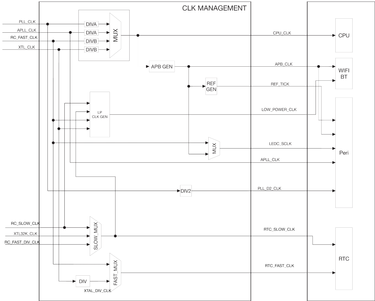
图 3-2. 系统时钟
