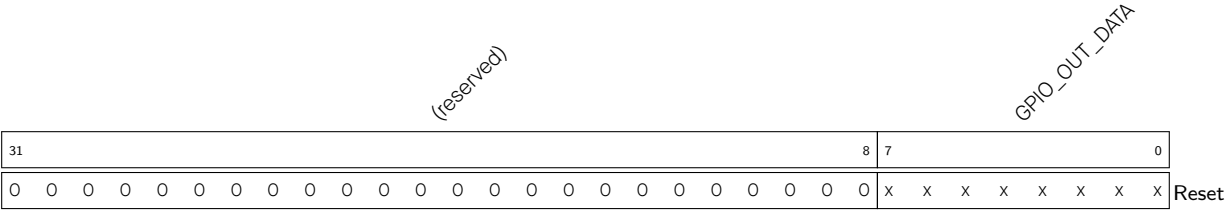
Register 4.5. GPIO_OUT1_WITS_REG (0x0014)
