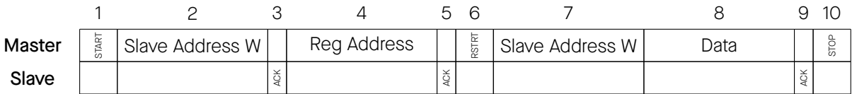
图 30-22. I²C 写操作
