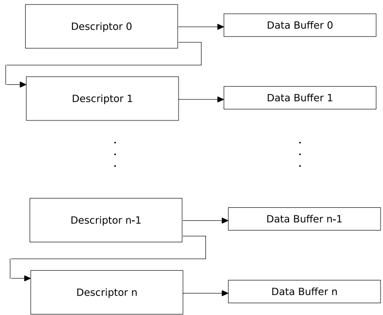
图 8-5. 链表串
