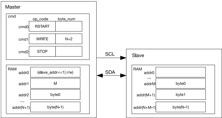
图 11-7. I2C Master 写 7-bit 地址 Slave 的 M 地址 RAM
