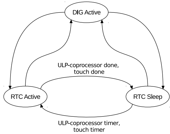
图 31-9. RTC 状态
