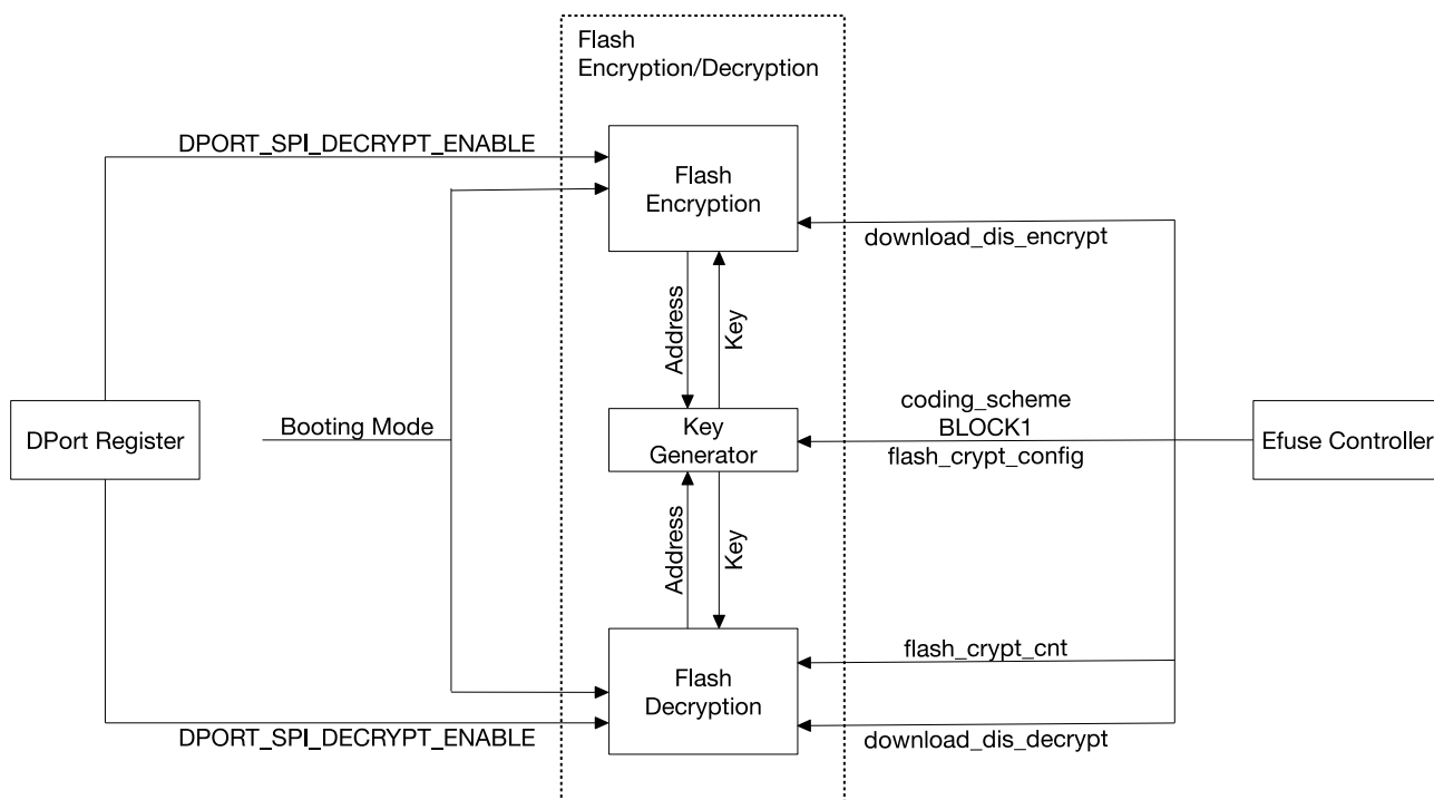
图 26-1. Flash 加解密模块架构
