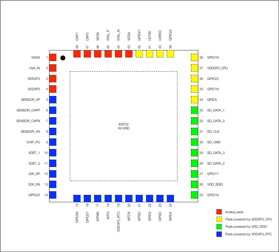
图 4-5. ESP32 I/O Pad 供电源 (QFN 5*5, 顶视图)
