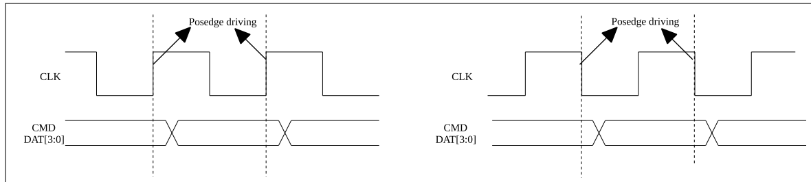
图 8-10. 输出时序图
