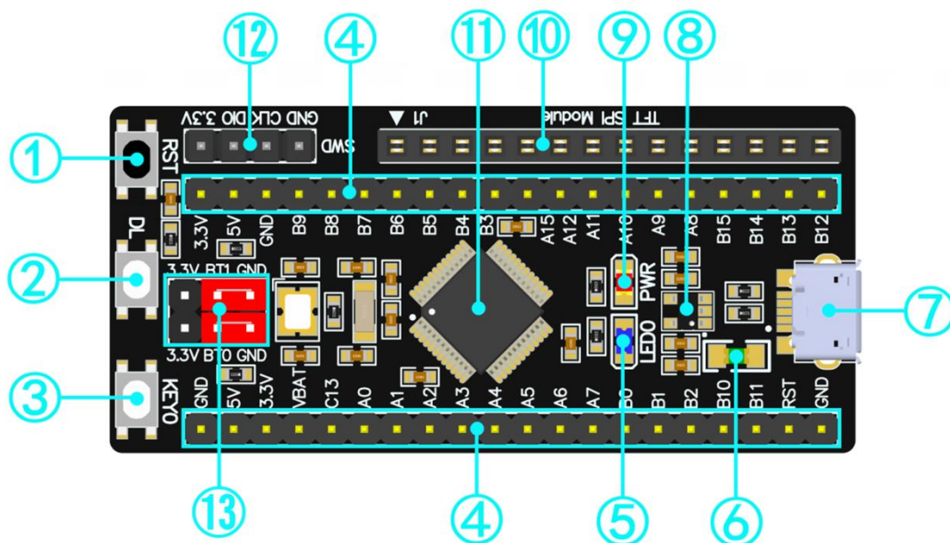
图 3. CH32F203C8T6 最小系统板硬件资源图
