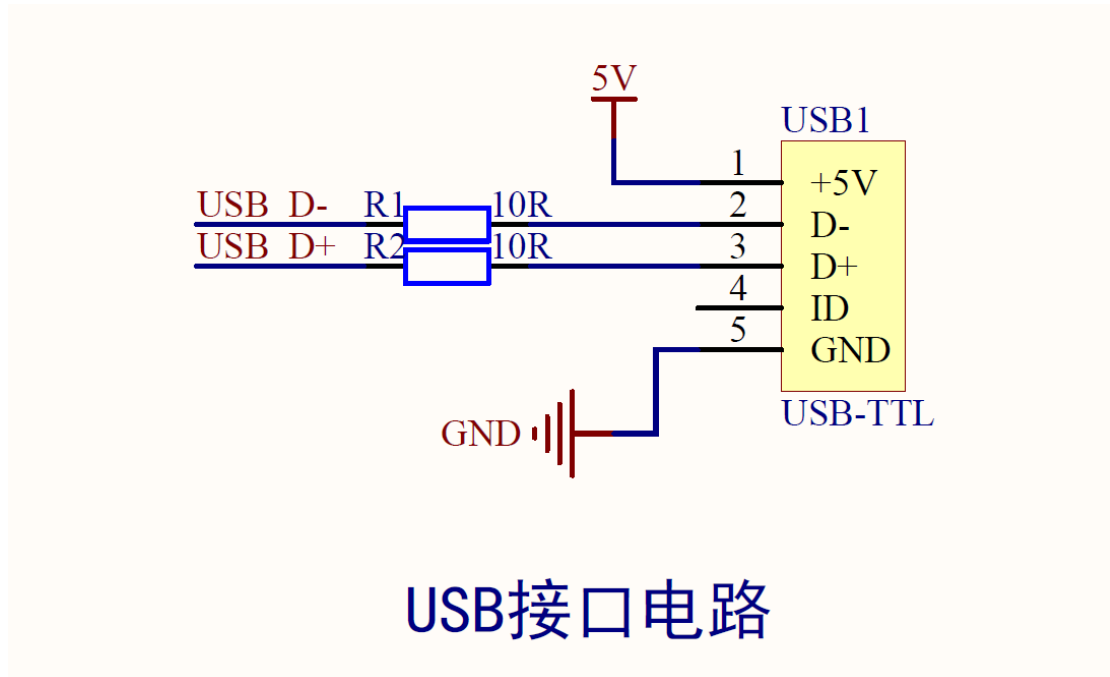
图 4. USB 接口原理图
