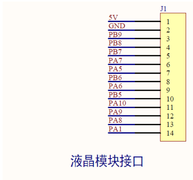
图 13. 液晶屏模块接口原理图
