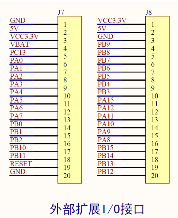
图 13. 外部扩展 I/O 接口
