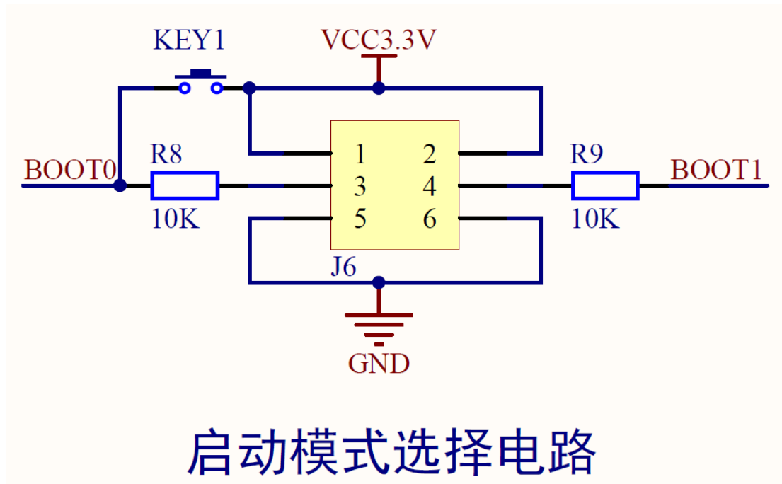
图 6. 启动模式选择原理图
