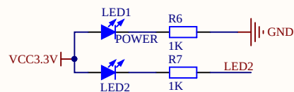
B 灯控制电路
