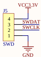
B 接口电路
