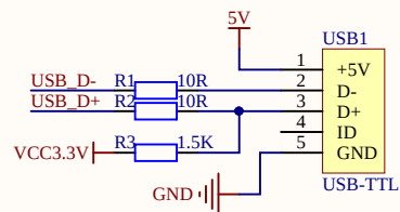
B 接口电路
