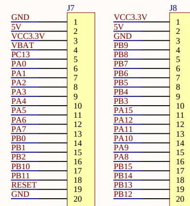
外部扩展 接口
