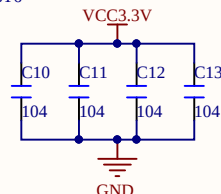
CH32F103C8T6主控电路
