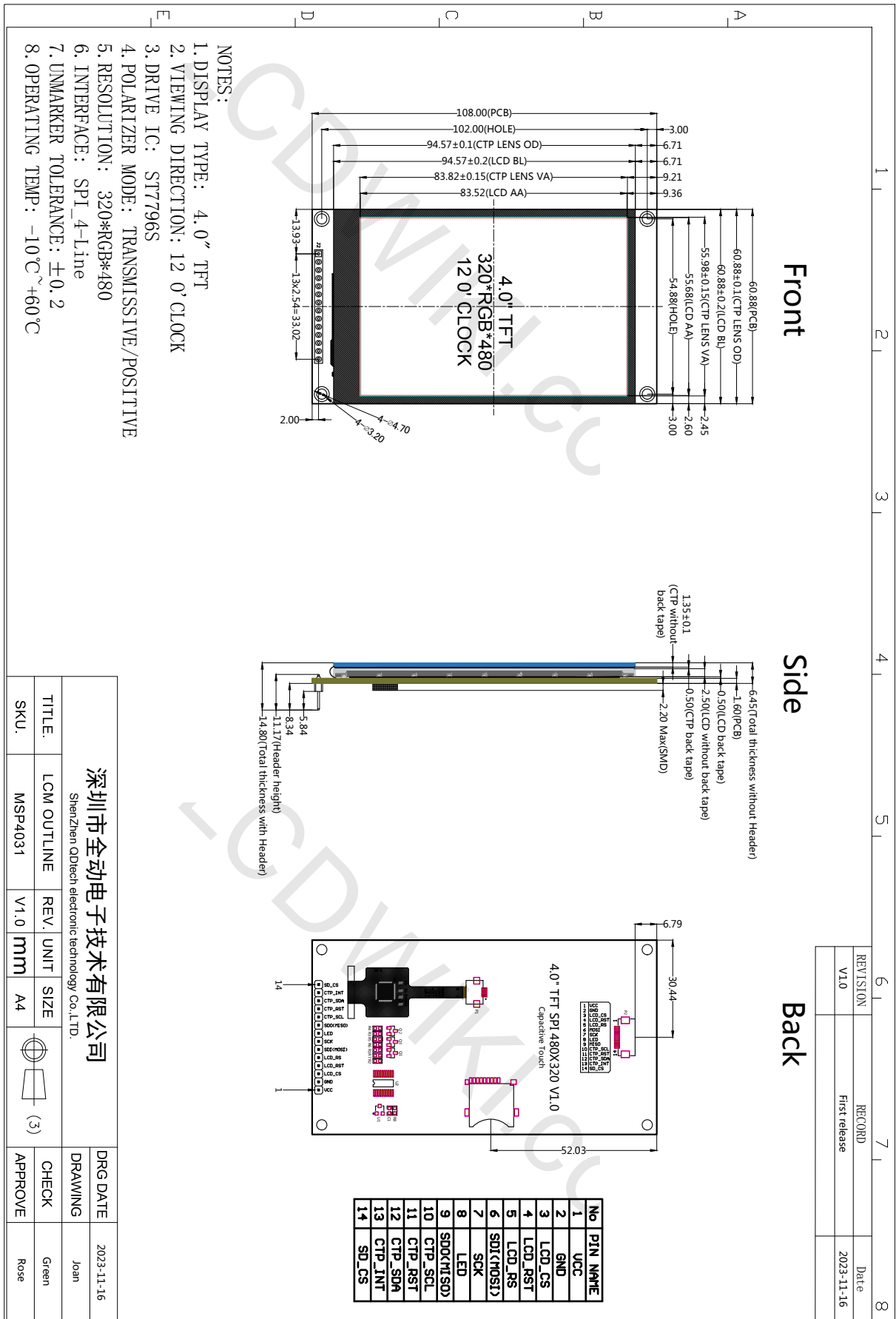
图 4 MSP4031尺寸图
