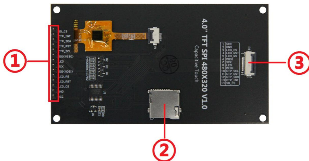
图 6 产品接口图
