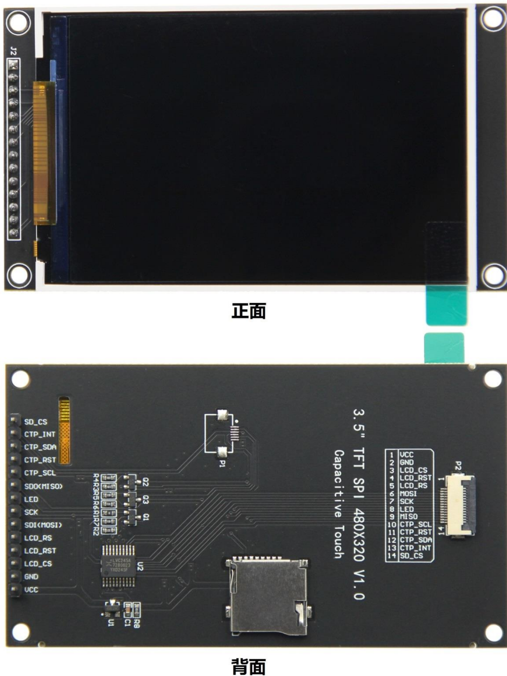
图 2 MSP3525（无触摸屏）产品图
