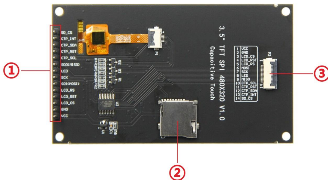
图 4 产品接口图
