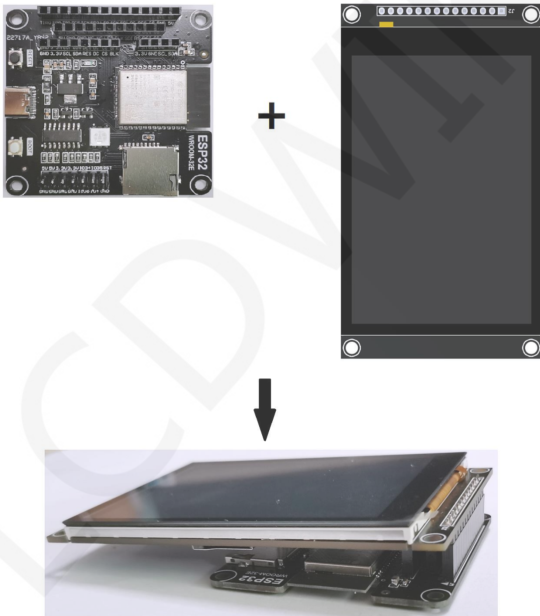
图1 模块直插ESP32-32E开发板
