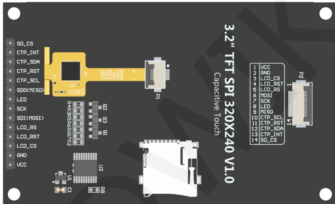
模块背面引脚
