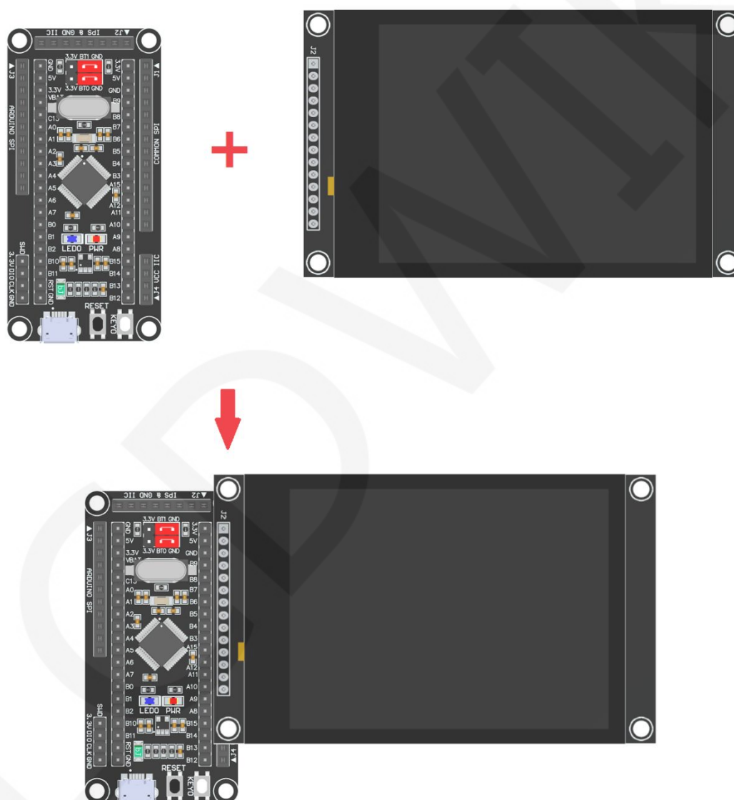
图1 模块直插CH32F103C8T6开发板
