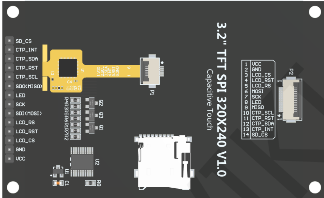
图3 模块背面引脚
