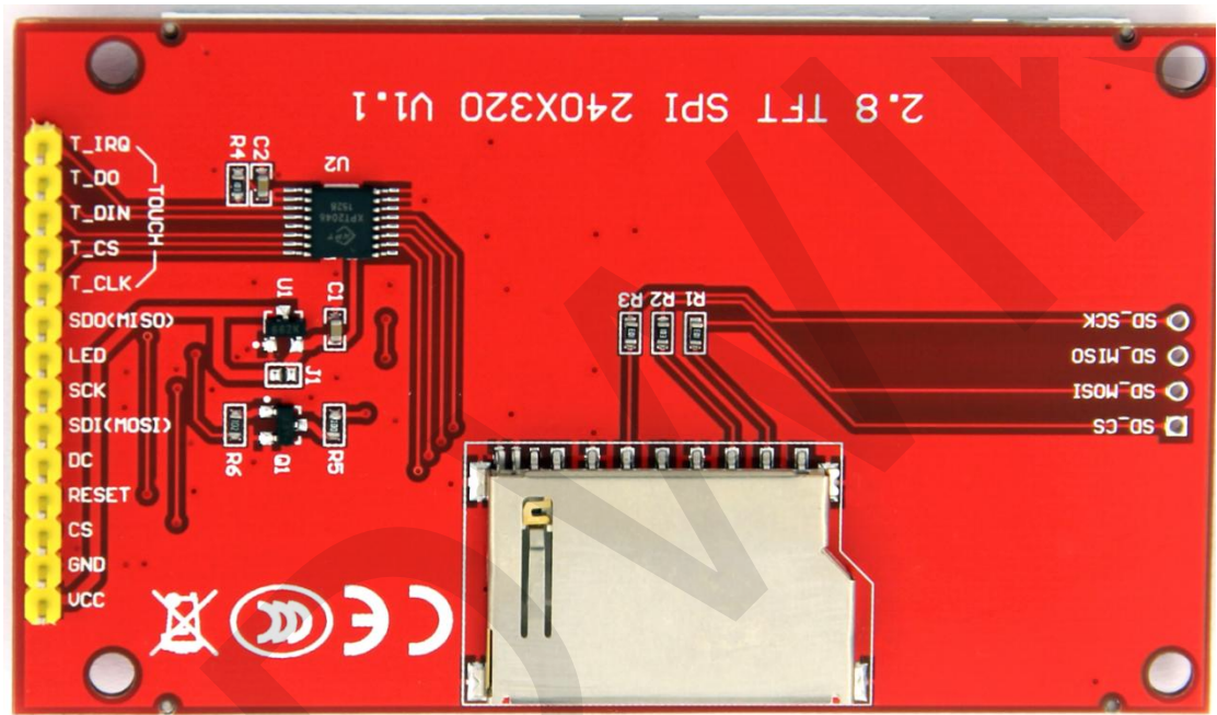
引脚丝印图
