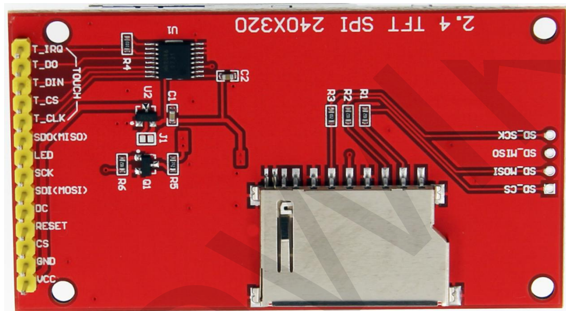
引脚丝印图
