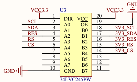
5V转3.3V电平转换电路
