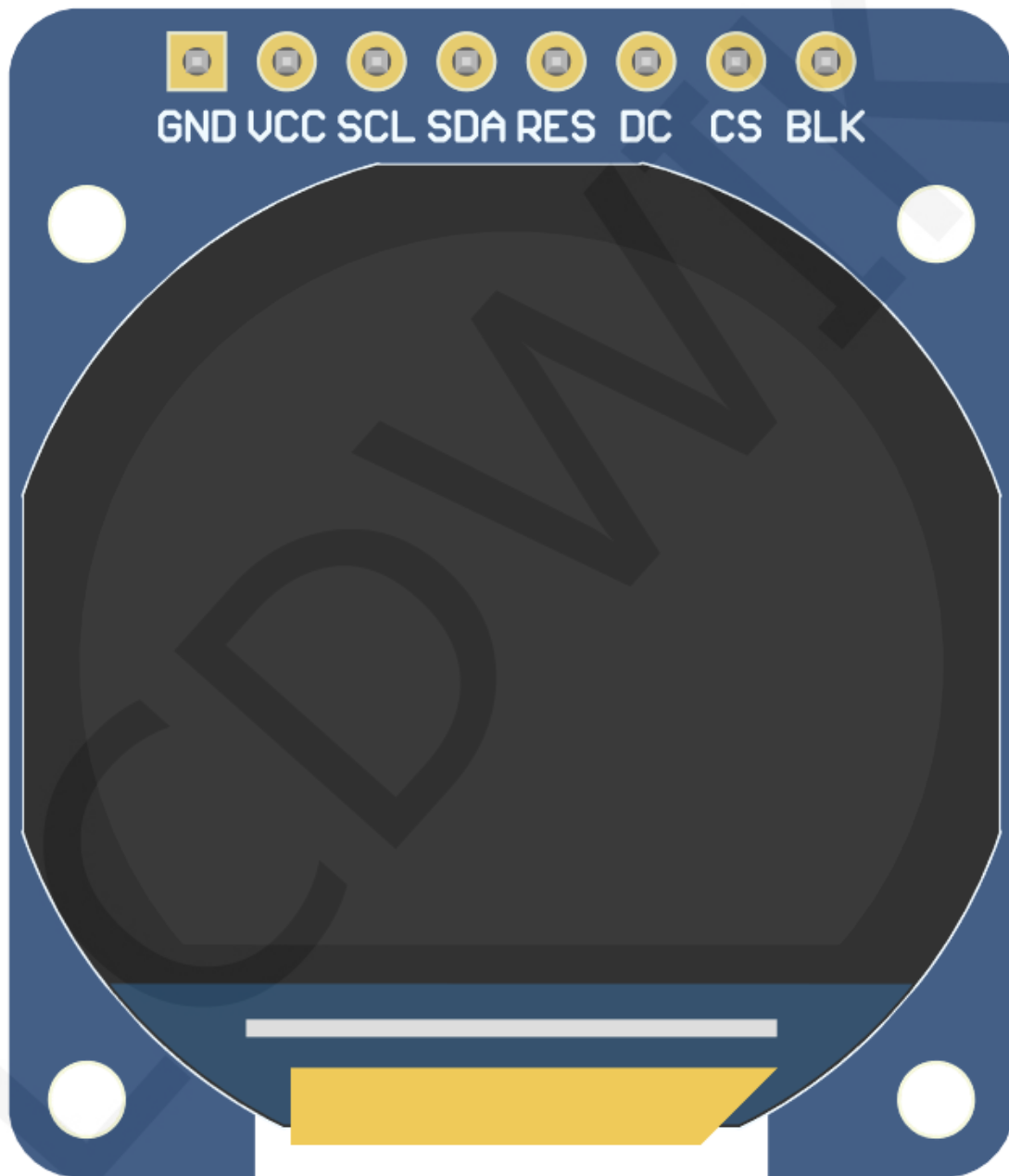
图1. 模块正面引脚图
