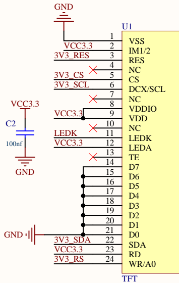
0.96寸IPS圆屏24Pin接口
