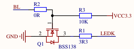
背光控制电路 (可IO或者PWM控制)
