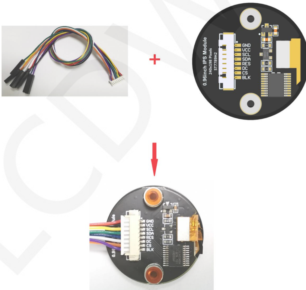
Picture1. Module wiring
