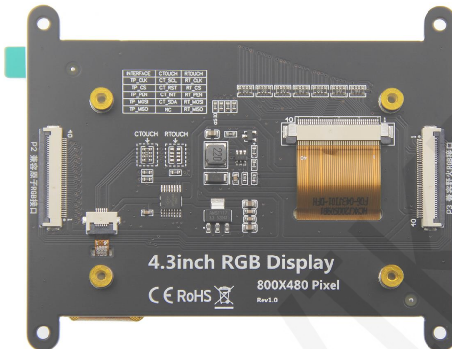
图 2. 模块背面图
