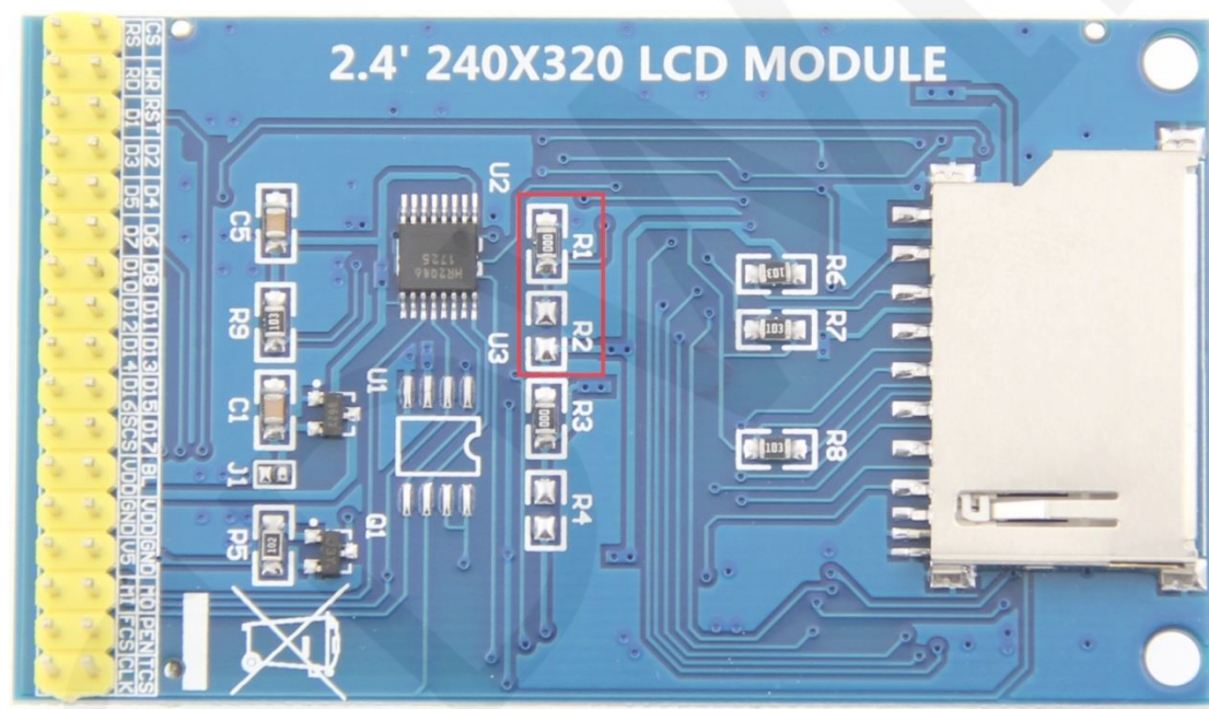
图 1. 模块引脚丝印图
