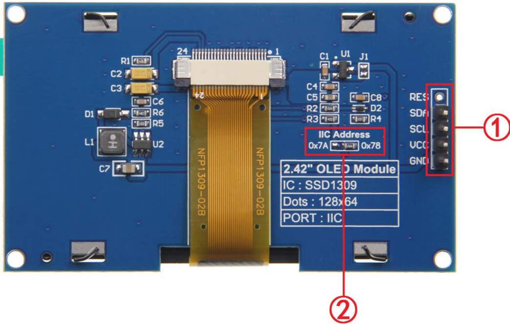
图 3 产品接口图
