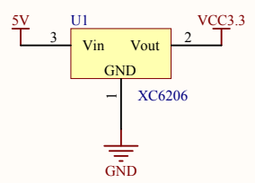
5V转3.3V电路
