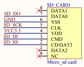
SD卡扩展接口电路
