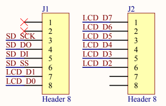
Arduino排针接口电路
