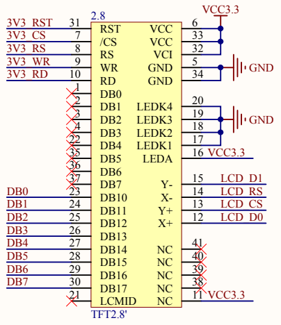
液晶屏37P接口电路
