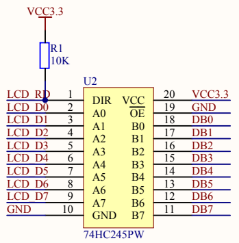
电平转换电路
