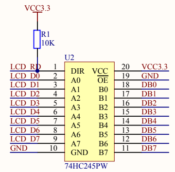
电平转换电路
