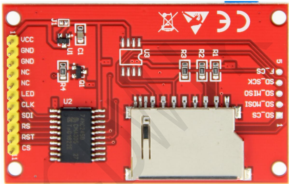
图1. 引脚丝印图
