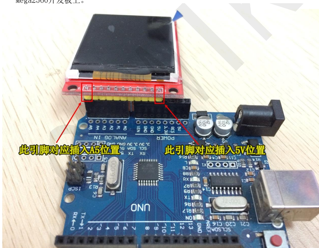
图2. 模块直插Arduino UNO图
