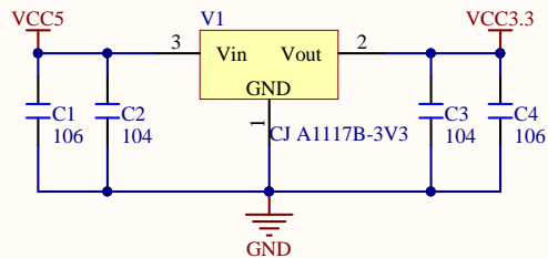
5V转3.3V稳压电路
