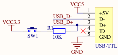
USB供电及下载电路
