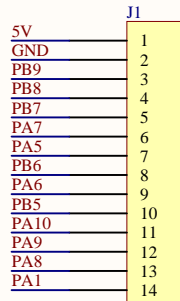
外部扩展I/O接口
