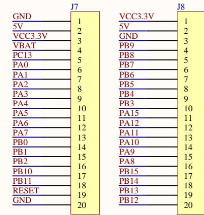
外部扩展I/O接口
