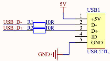
USB接口电路
